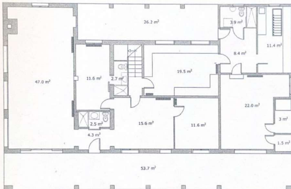
PLANTA BAIXA
