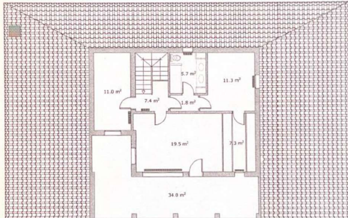
PLANTA PRIMERA
