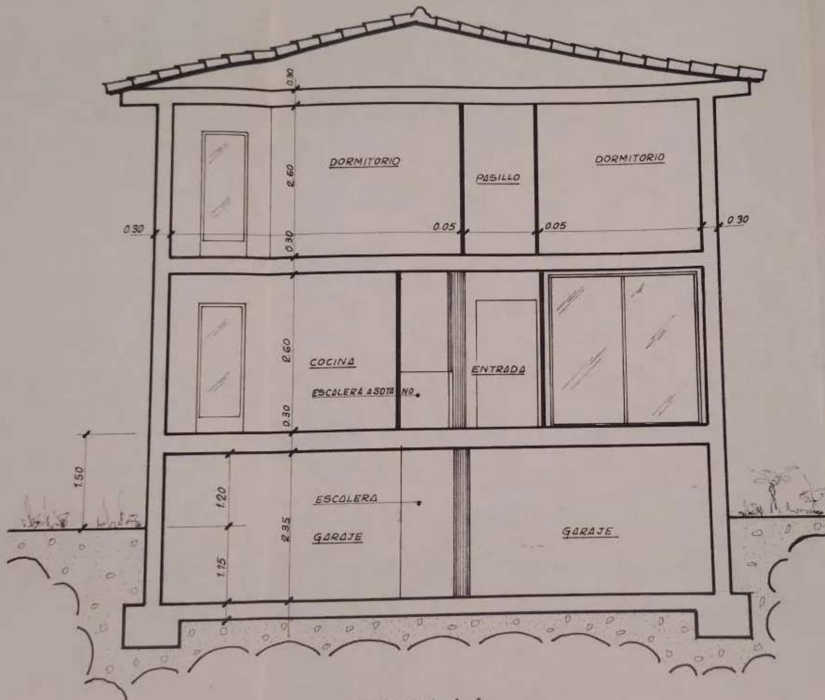
SECCION A-A.
