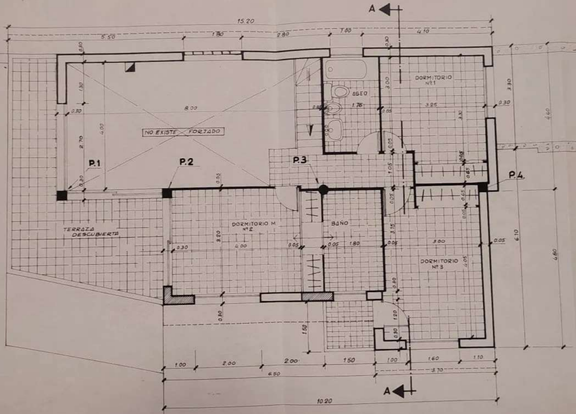
PLANTA PISO
