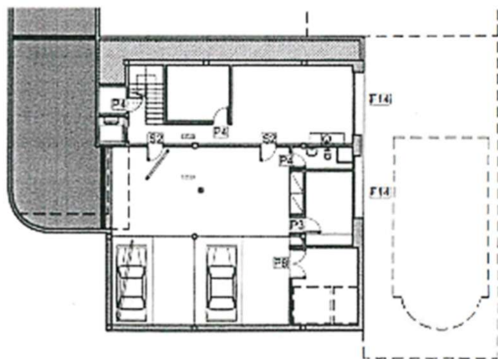
PLANTA SOTERRANI
