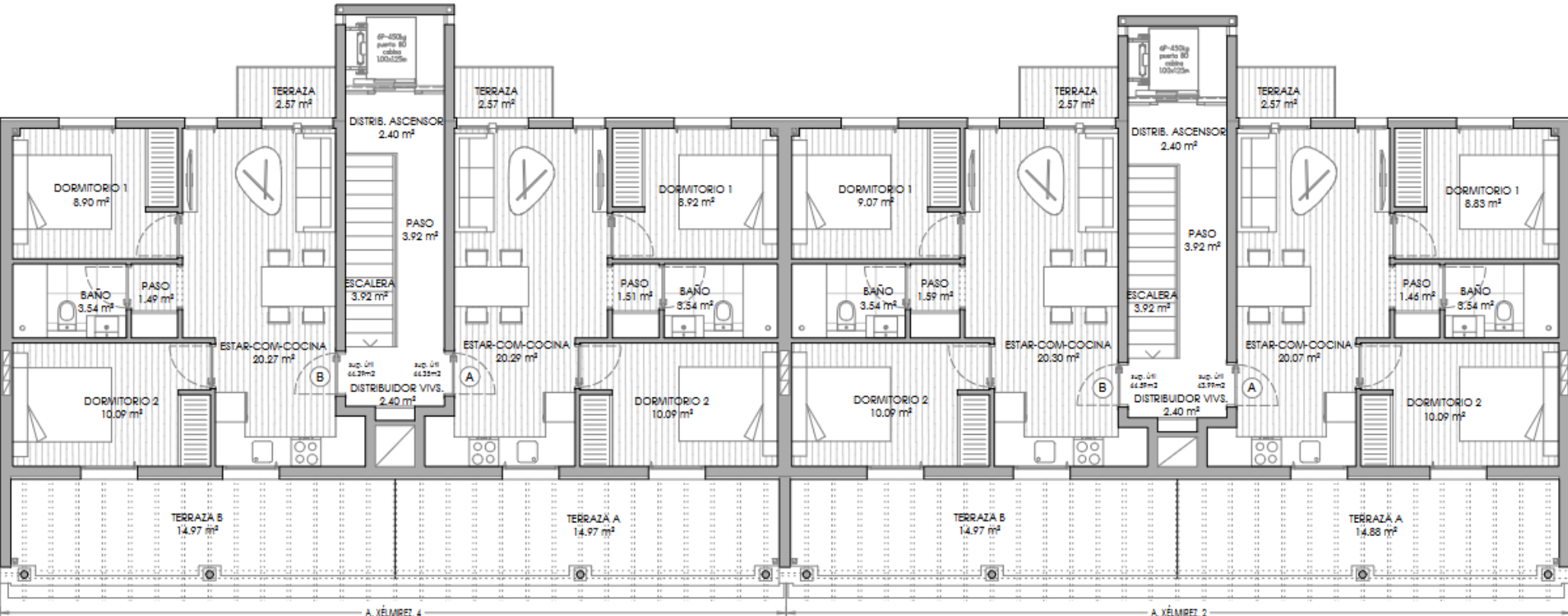
PLANTA 5ª Distribución
