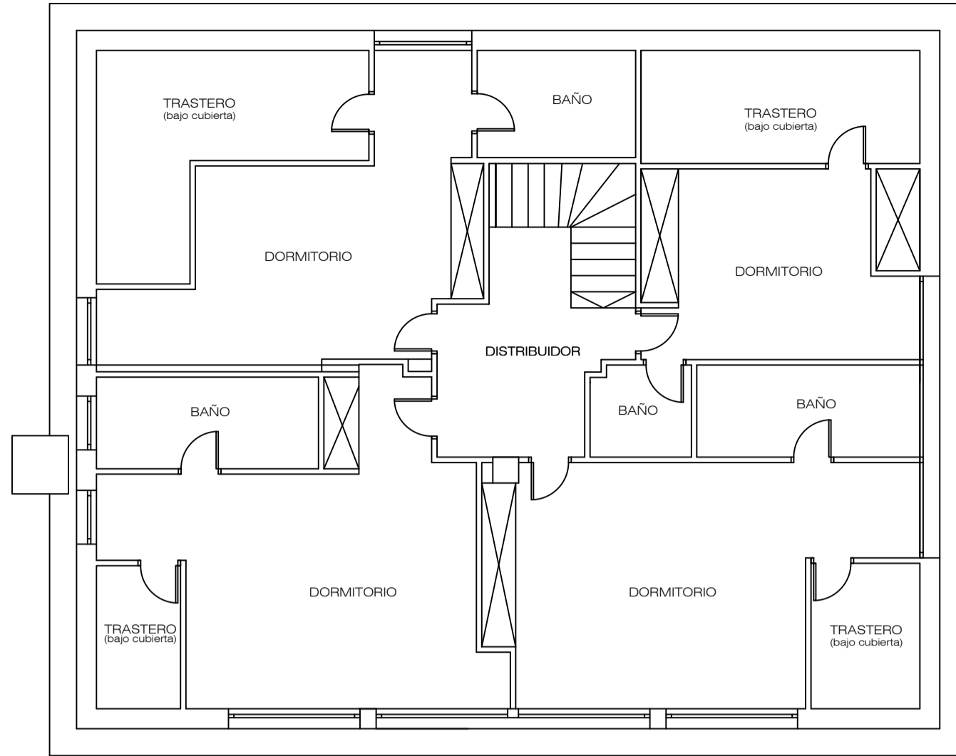
PLANTA SEGUNDA E:1/100
