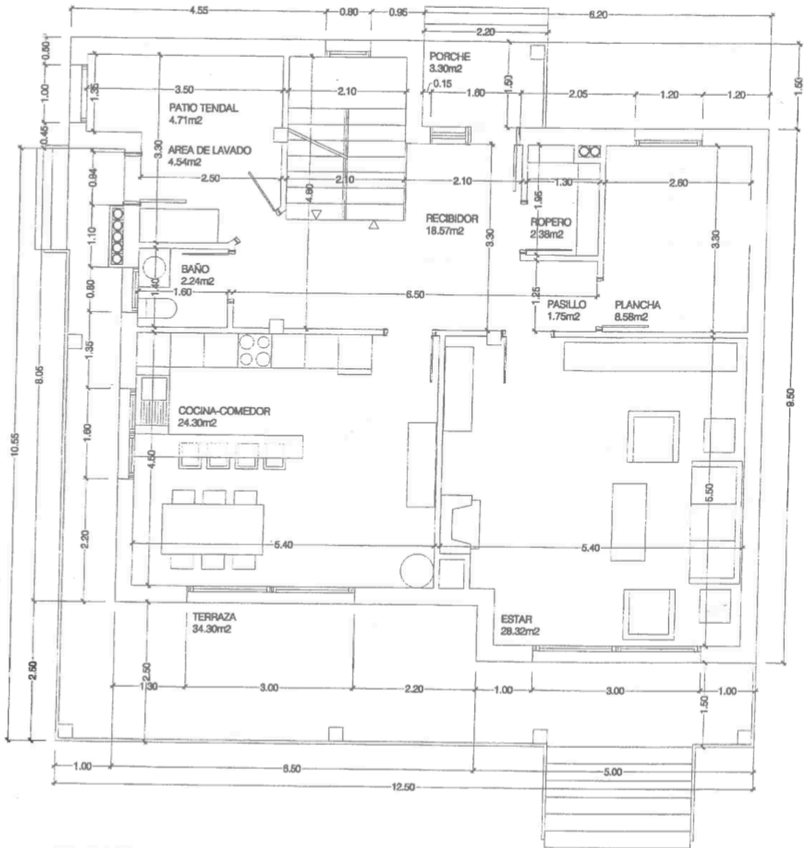
PLANTA BAJA
