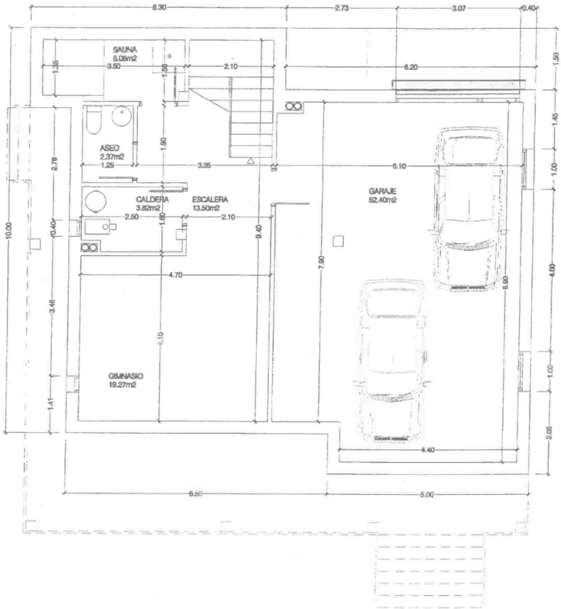
PLANTA SOTANO
