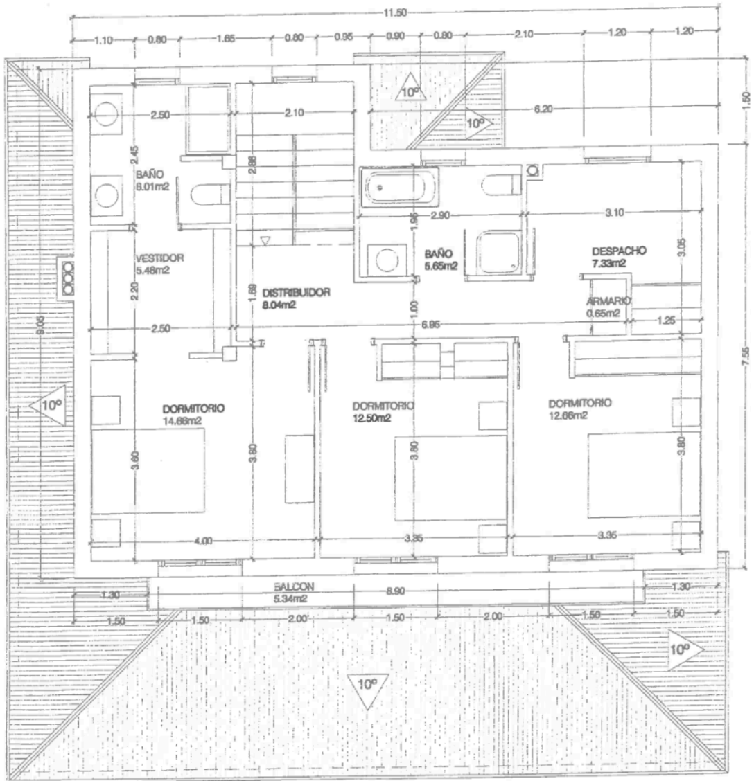
PLANTA PISO
