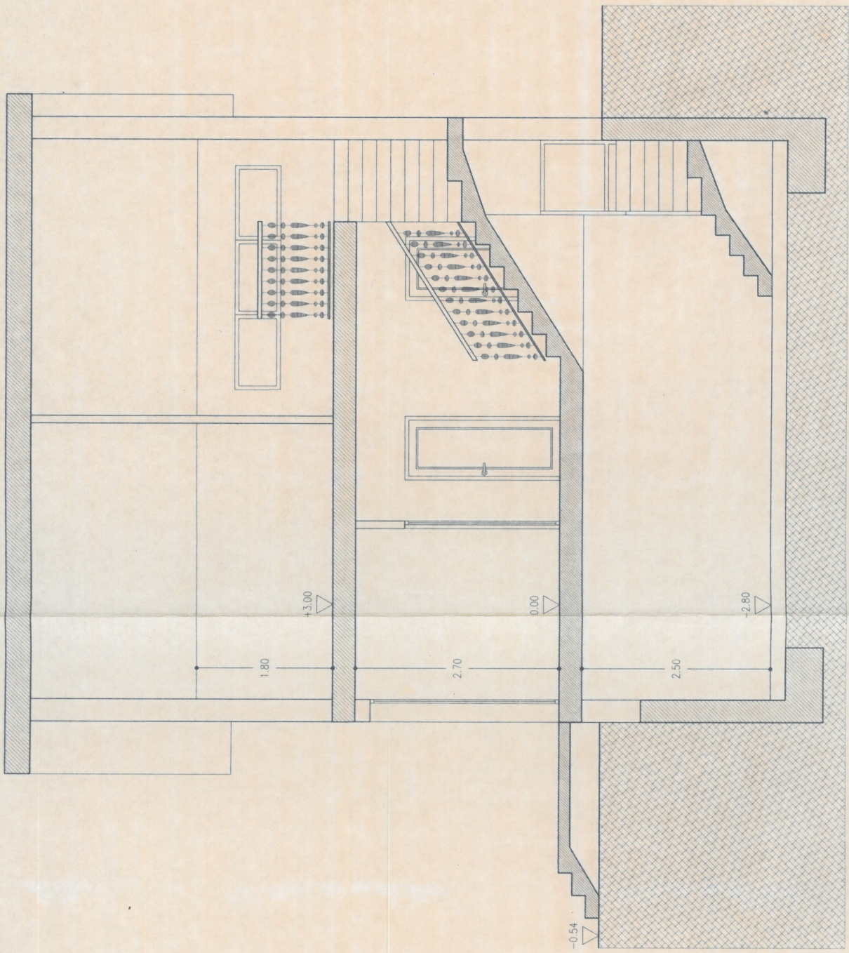
SECCION A-A
