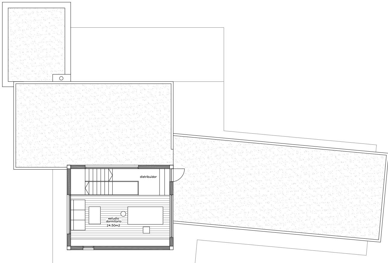
PLANTA PRIMERA
