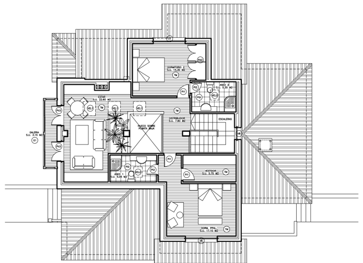
ARQUITECTURA Superficie Construida : 92.60 M 2
