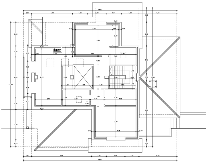
REPLANTEO Y COTAS
