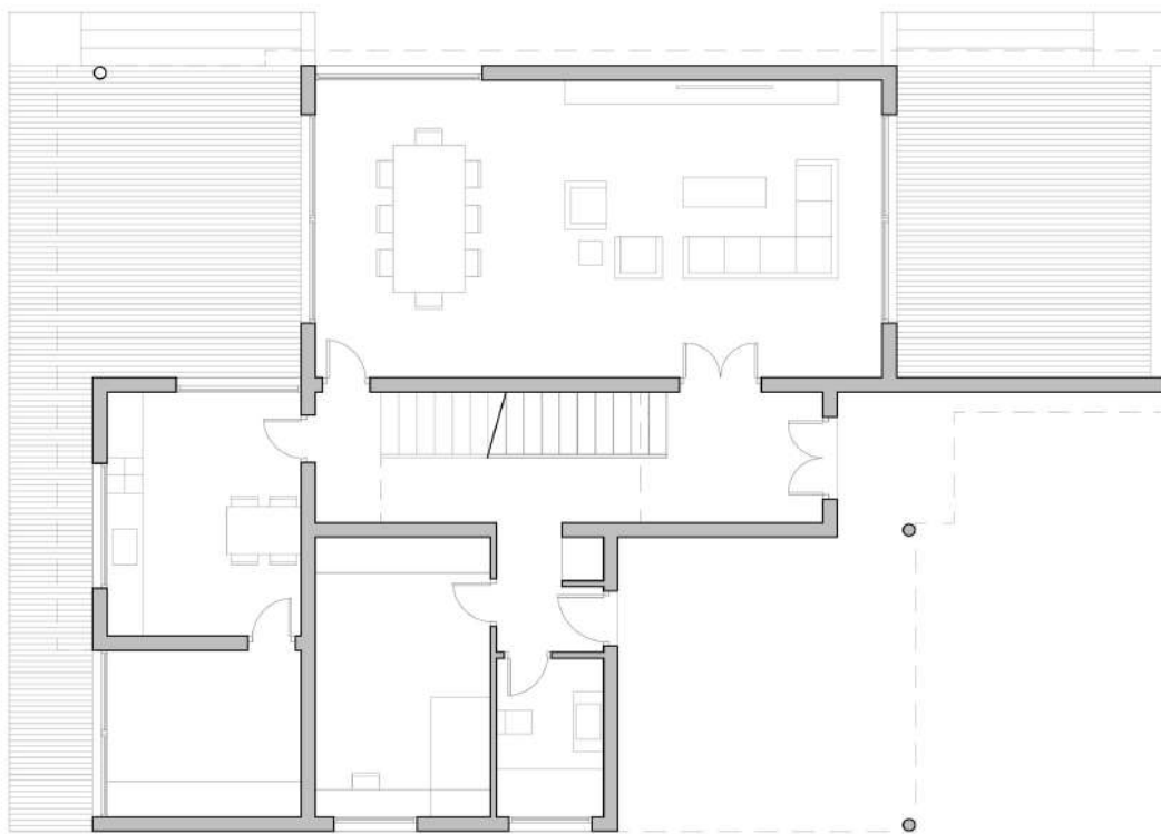
ESTADO ACTUAL PLANTA BAJA
