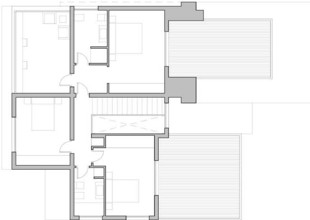
ESTADO ACTUAL PLANTA PRIMERA
