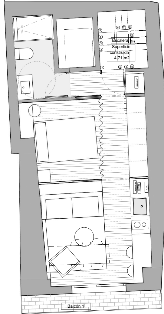
PLANTA SEGUNDA
