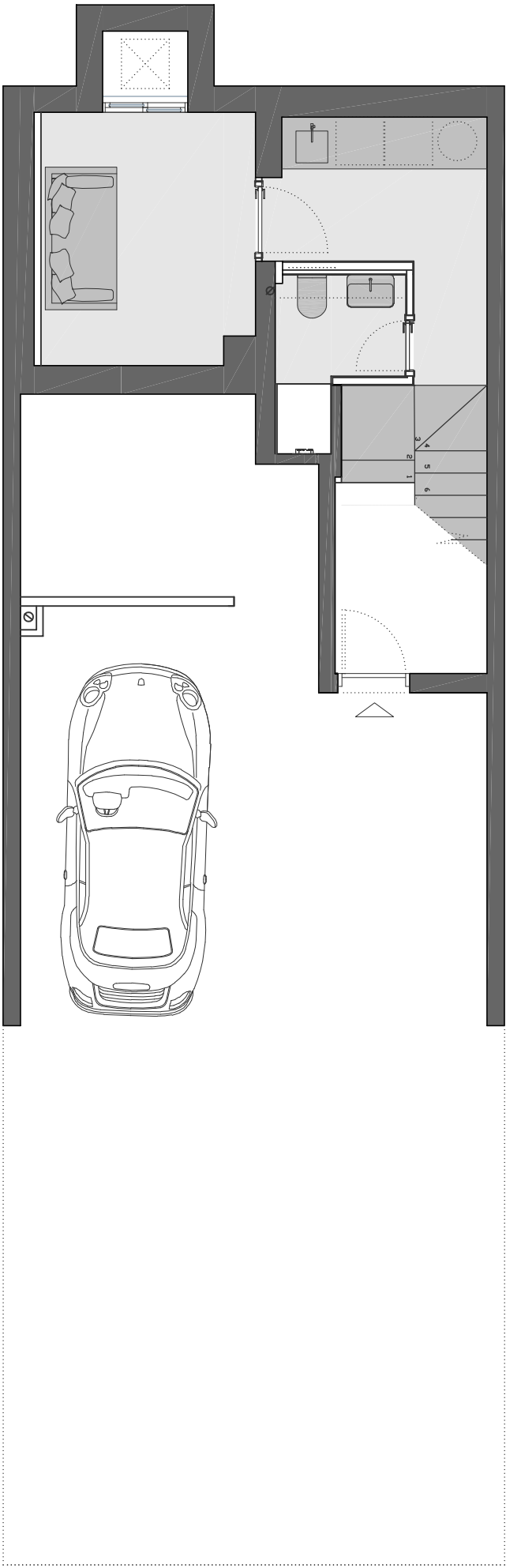
PLANTA SOTANO
