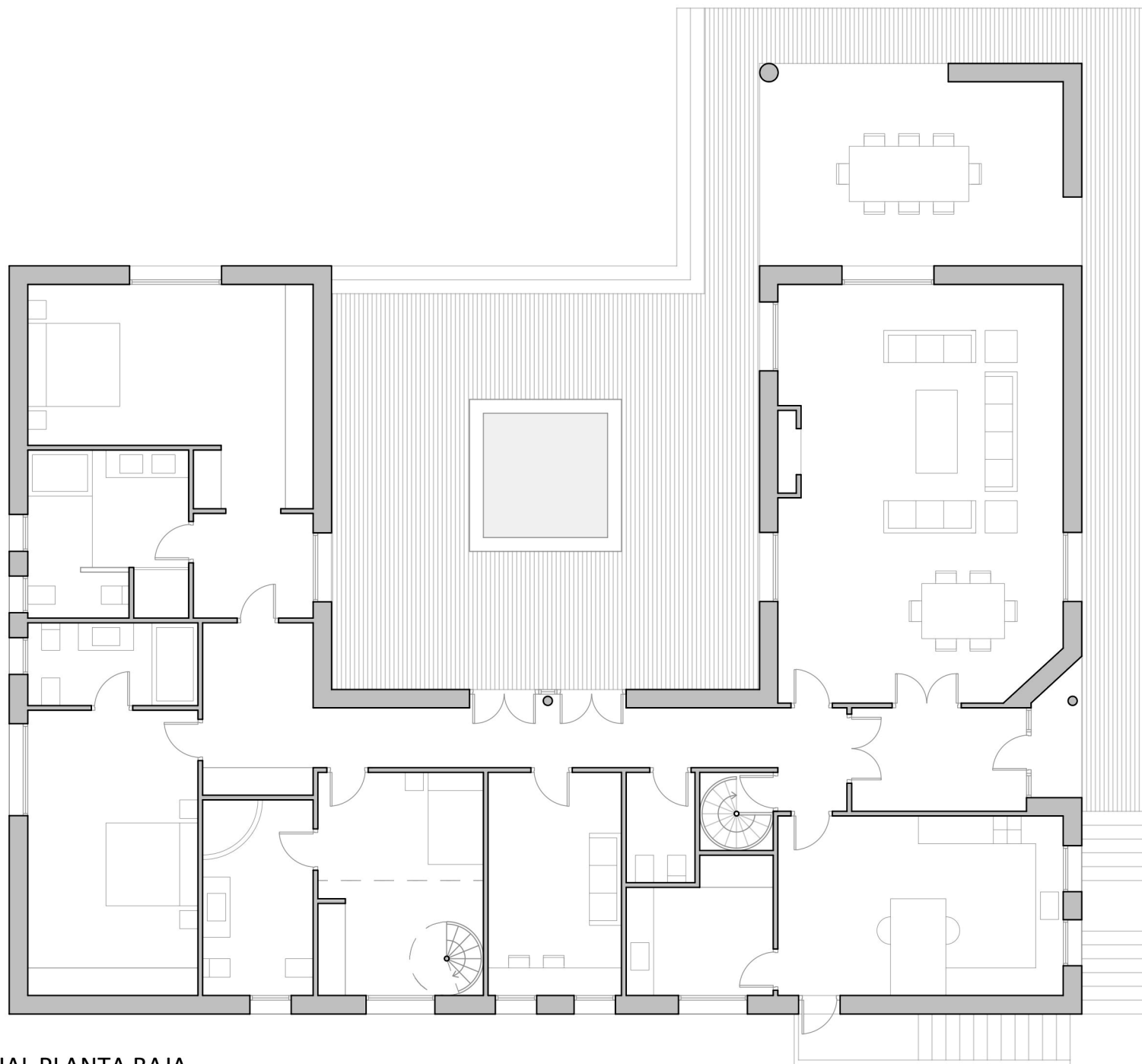
ESTADO ACTUAL PLANTA BAJA
