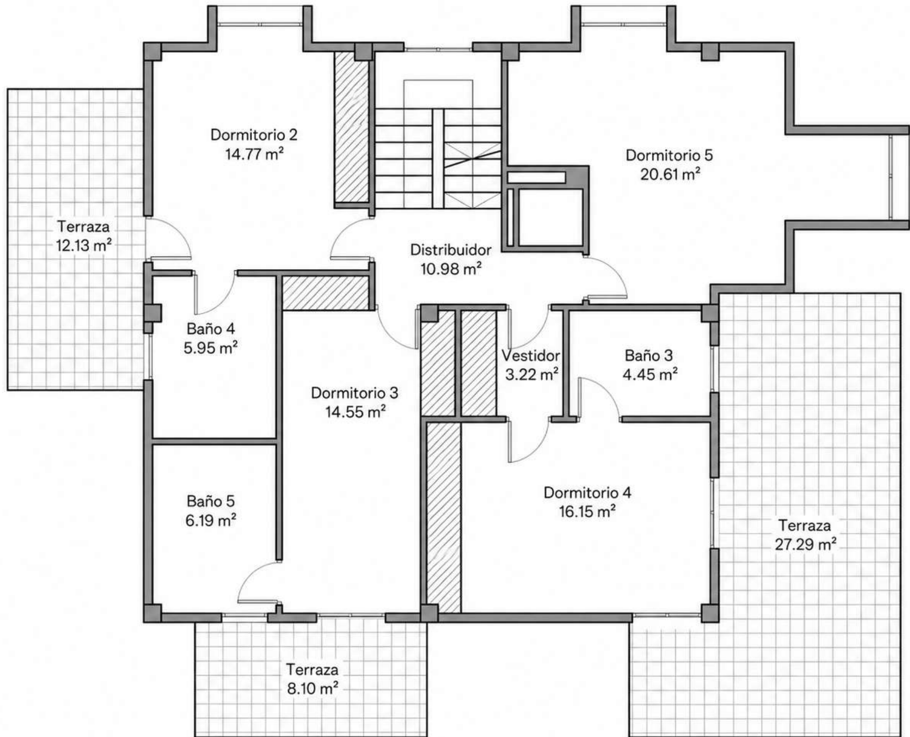
PLANTA PRIMERA
