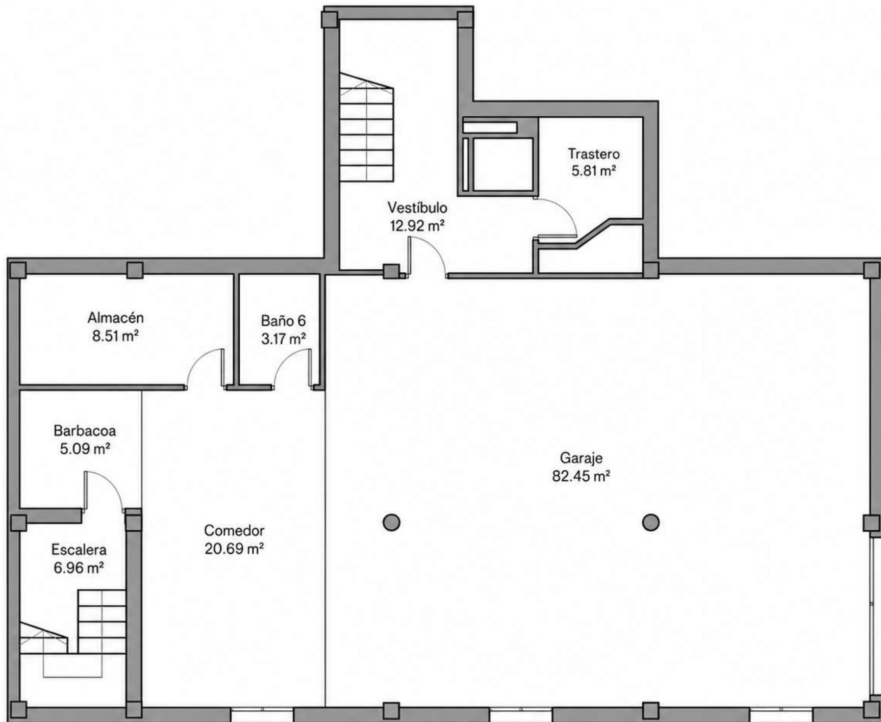
PLANTA SÓTANO
