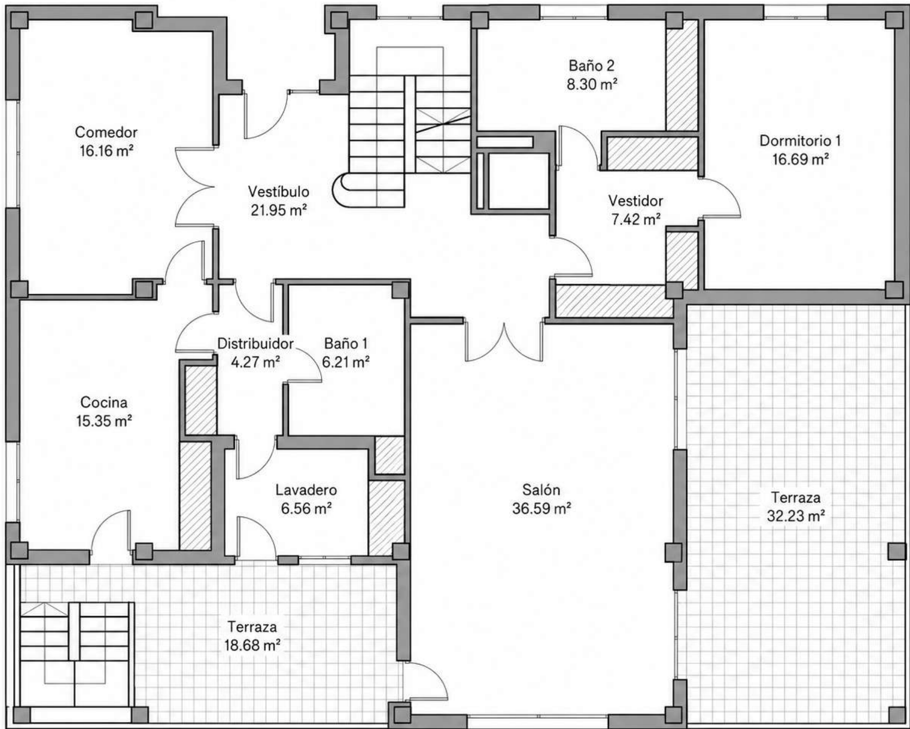
PLANTA BAJA
