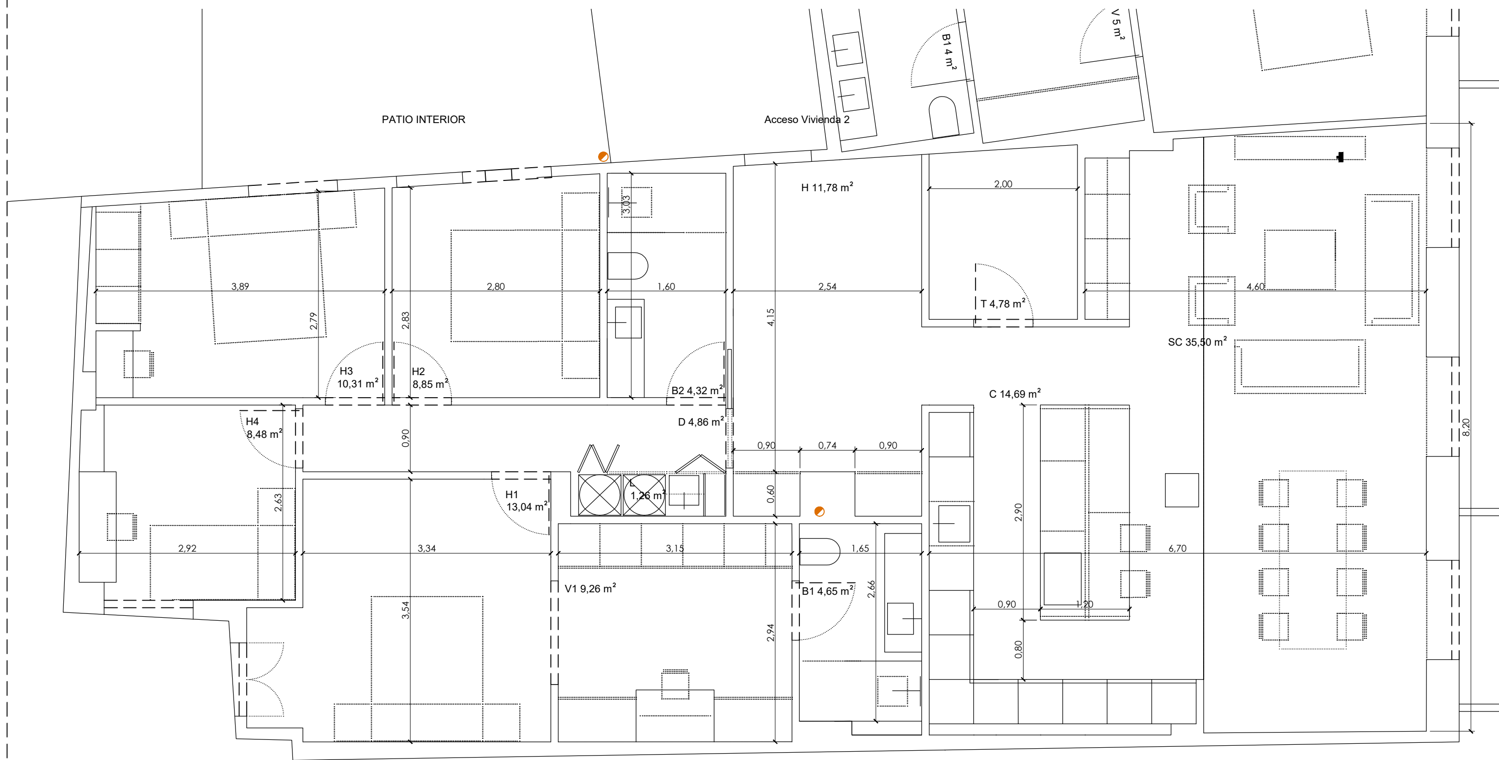
PLANTA E 1:50
