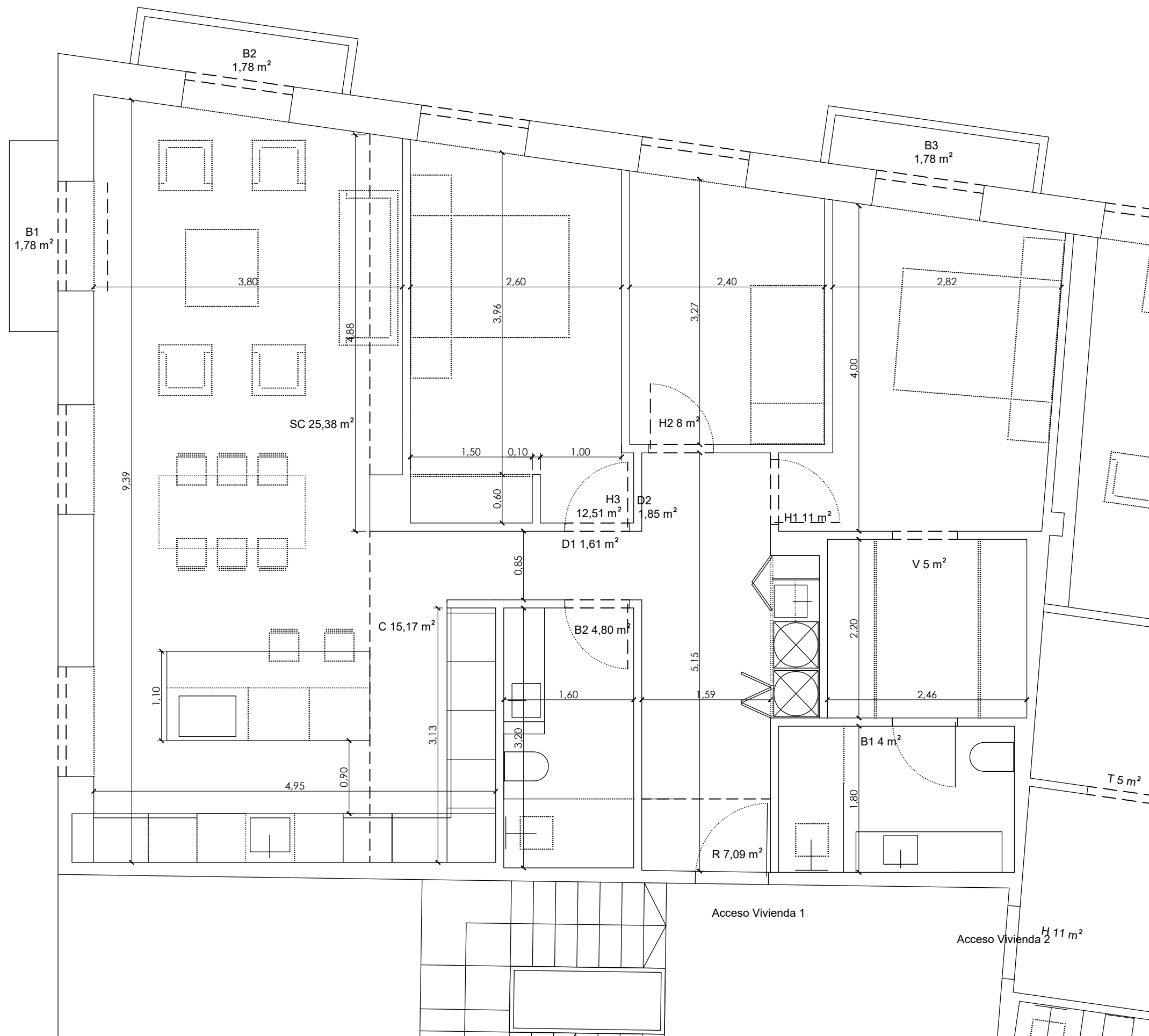
PLANTA E 1:50
