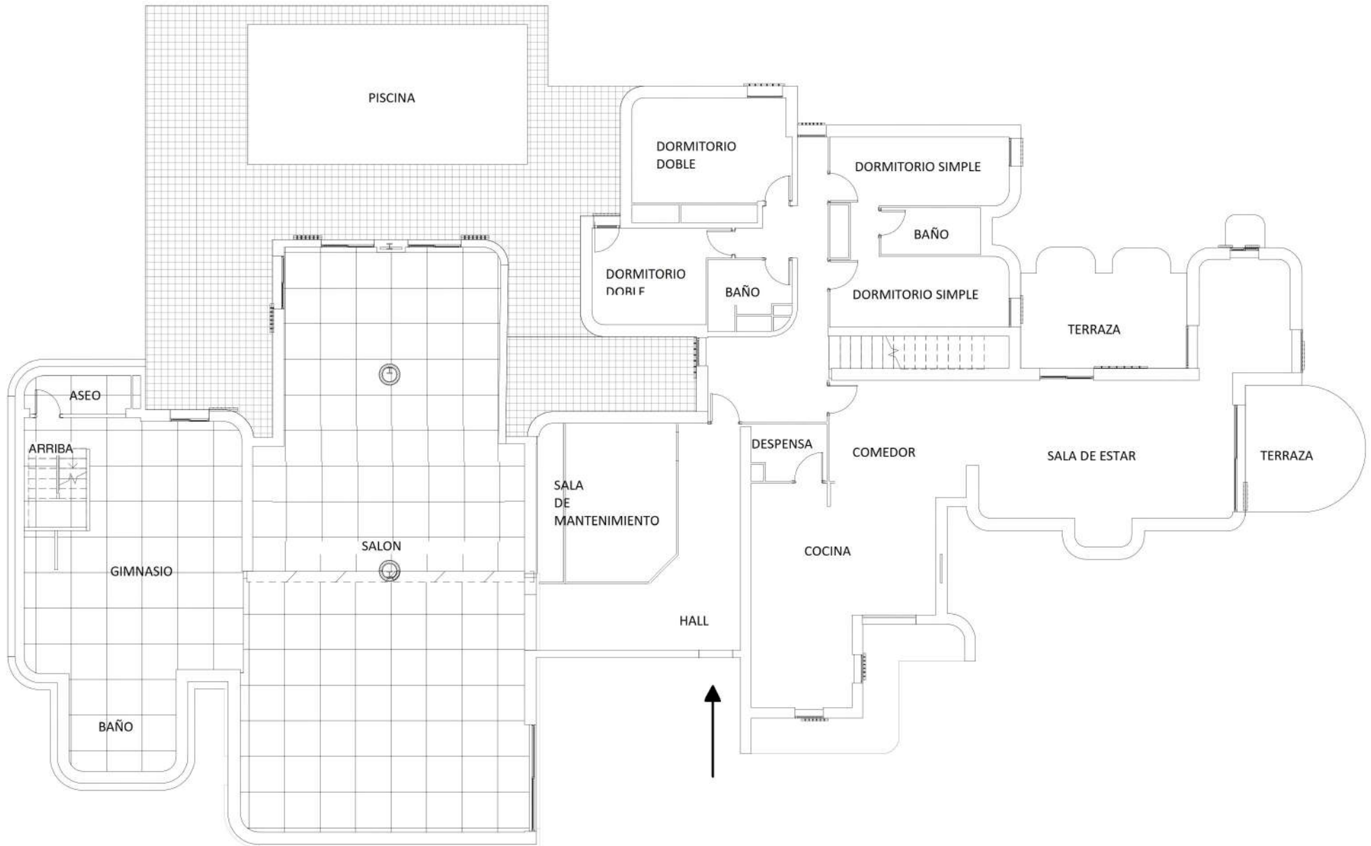
PLANTA BAJA
