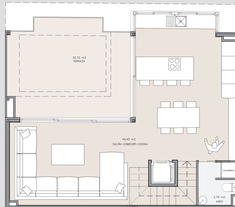
Planta Primera
