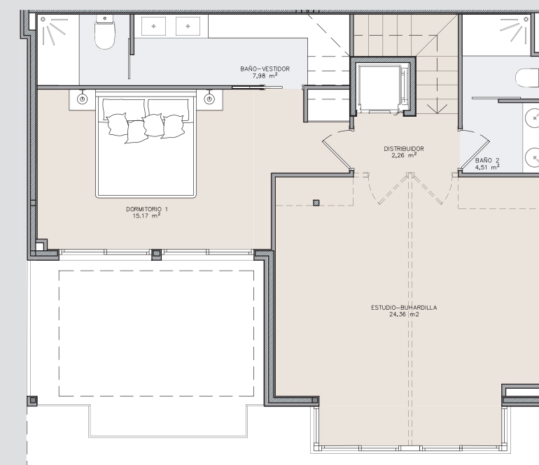
Planta Segunda
