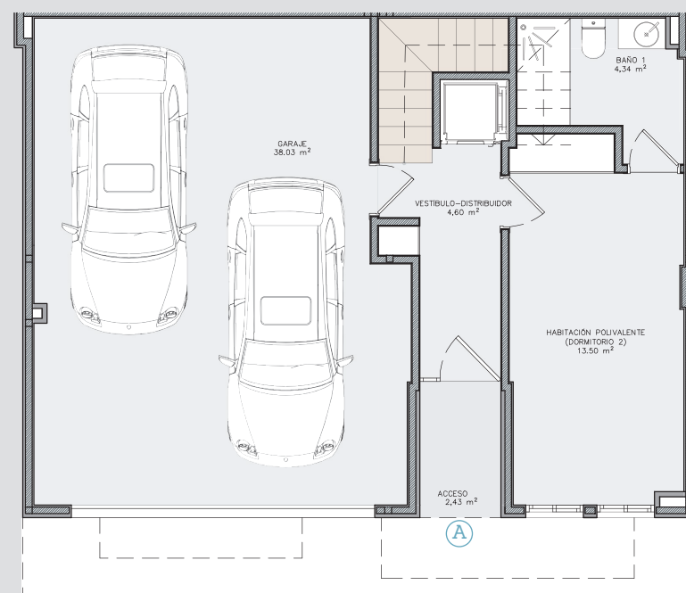
Planta Baja
