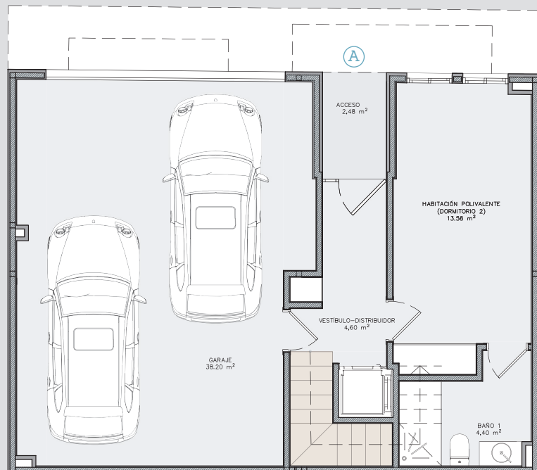
Planta Baja
