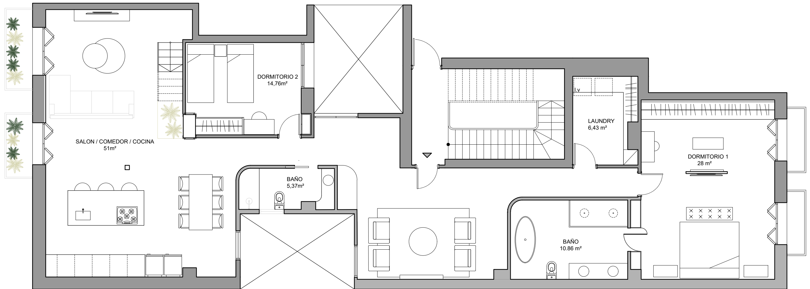
PLANO DE DISTRIBUCIÓN ESC: 1/75
