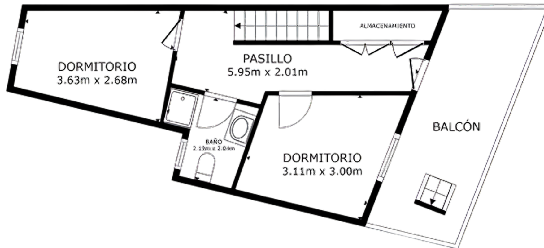
PLANTA 3
