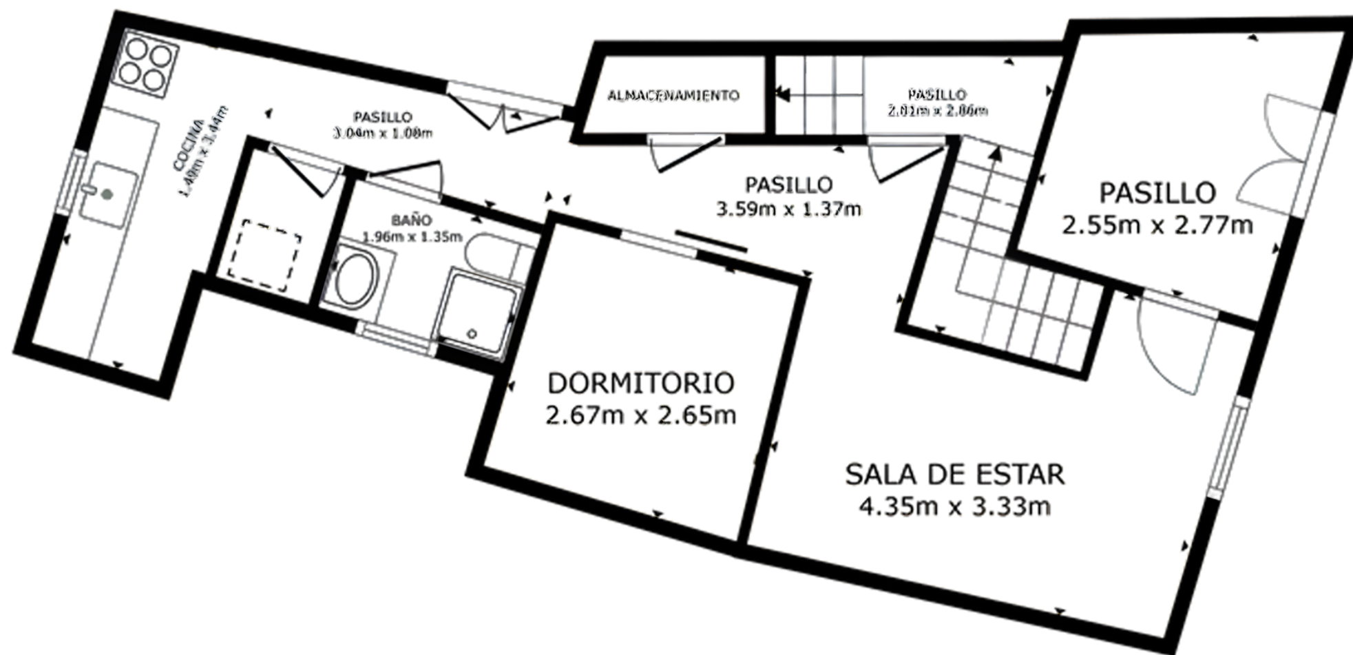
PLANTA 1
