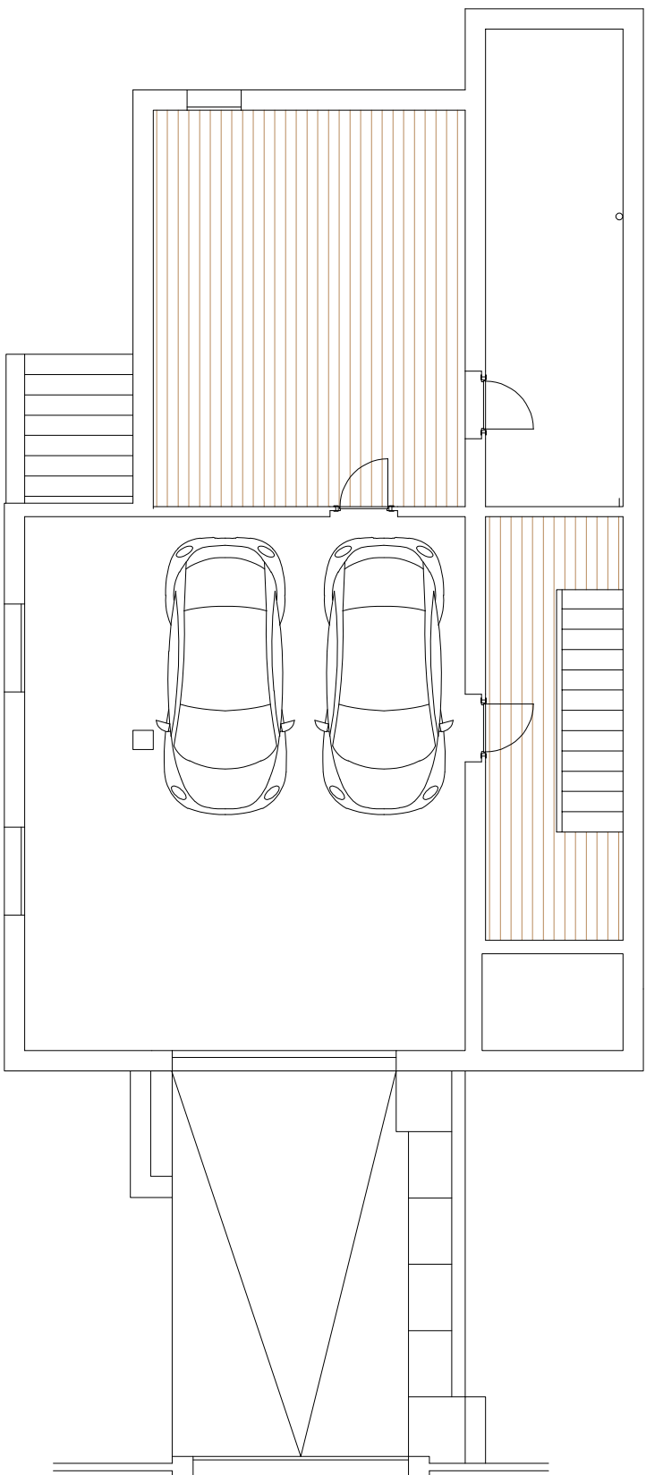
PLANTA SEMI-SOTERRANI
