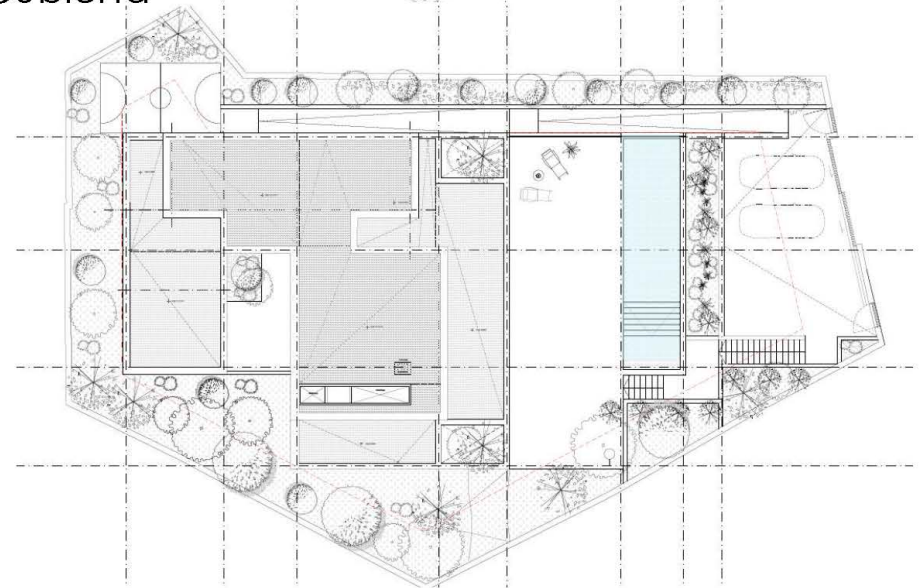
Planta Cubierta
