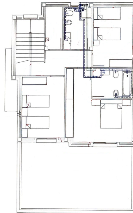
PLANTA PIS
