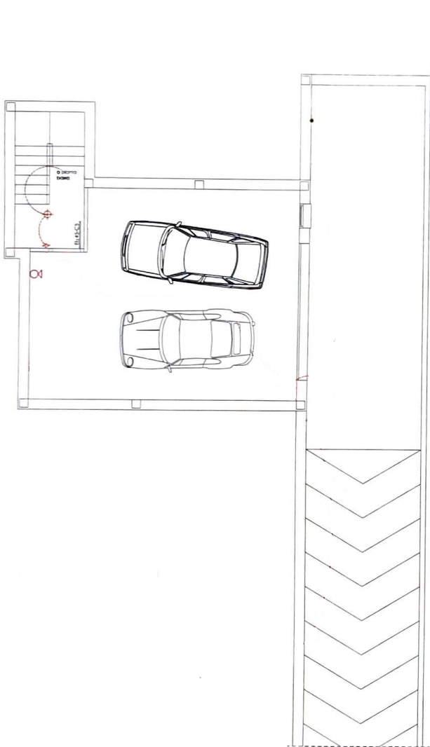
PLANTA SOTERRANI
