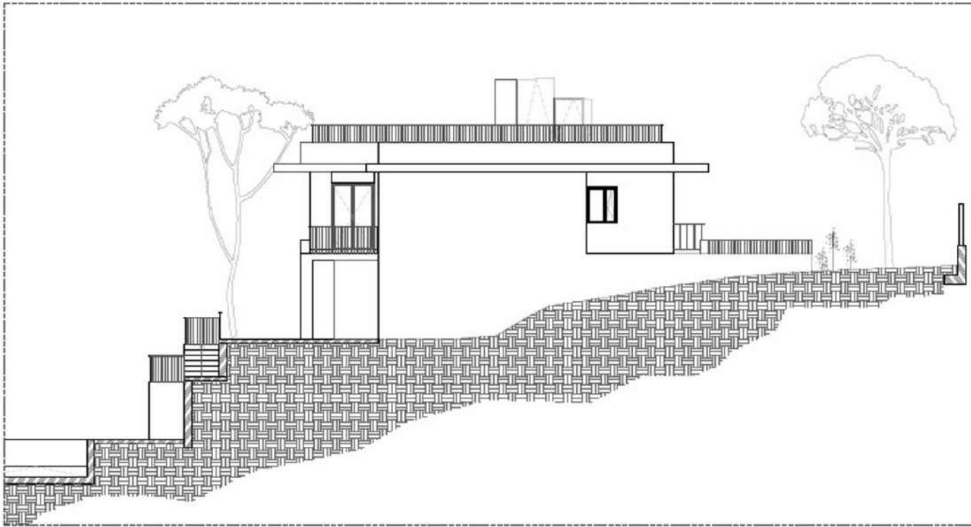
ALZADO OESTE
