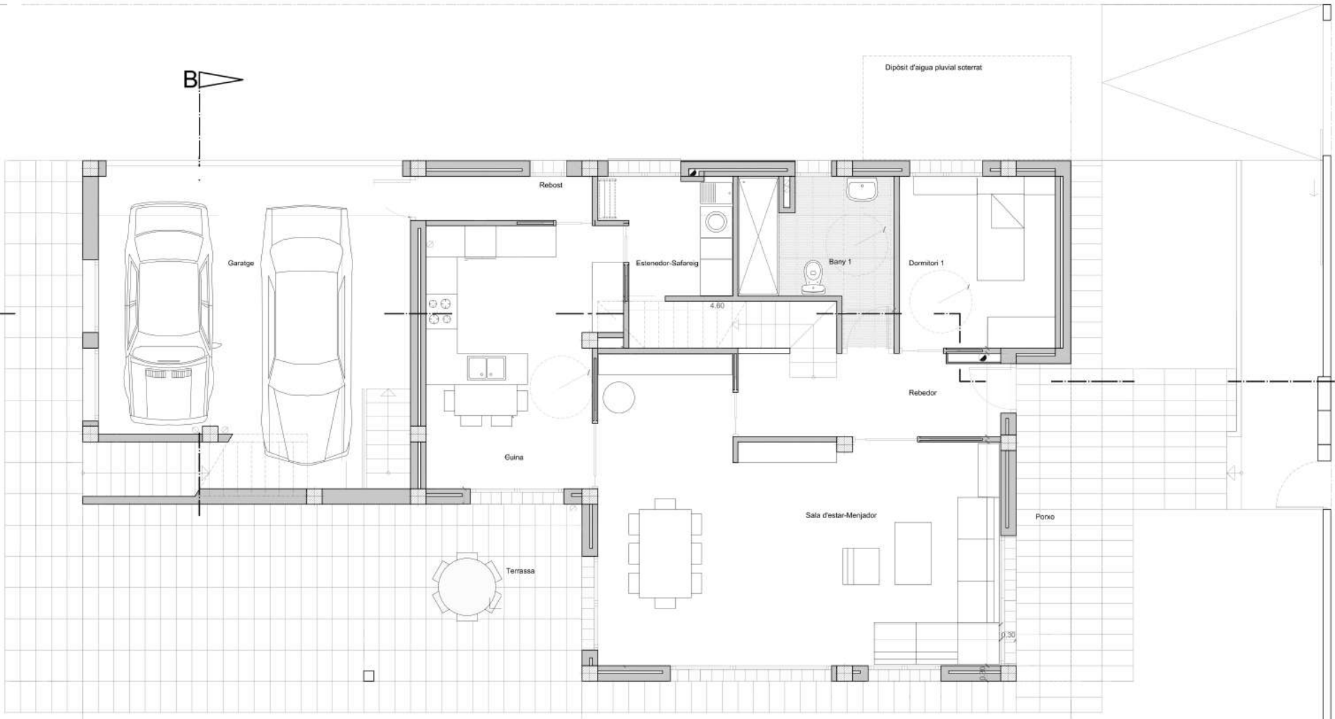
PLANTA BAIXA
