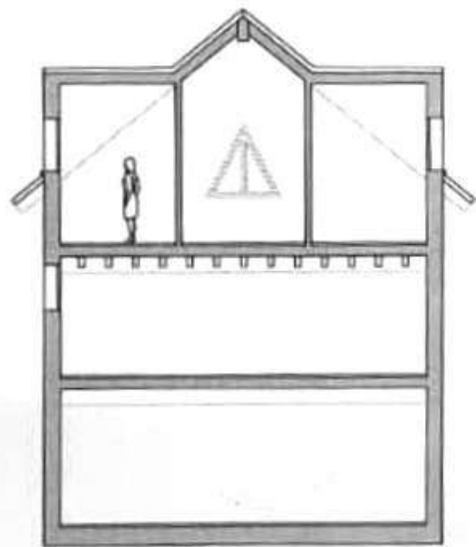
SECCO TRANSVERSA
