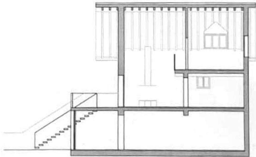
SECCO LONGITUDINAL
