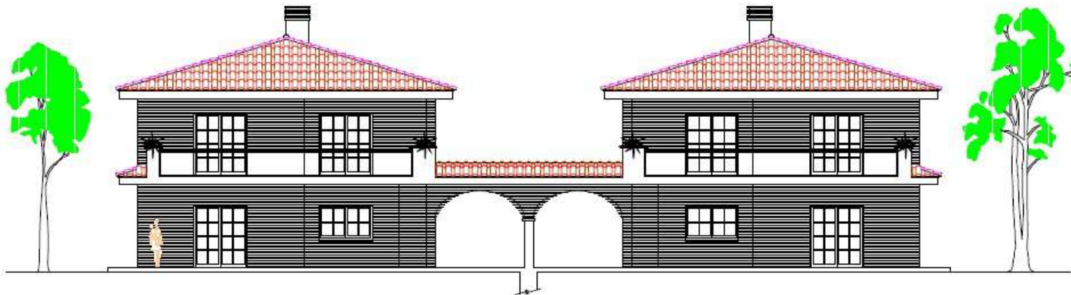
FACHADA POSTERIOR S.E.
