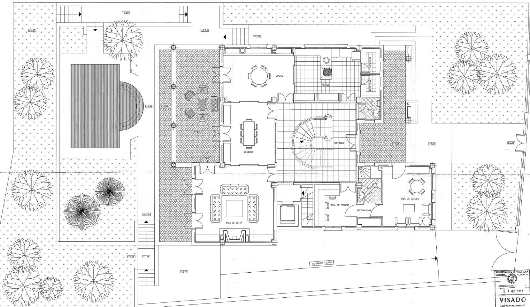
PLANTA BAJA.-
