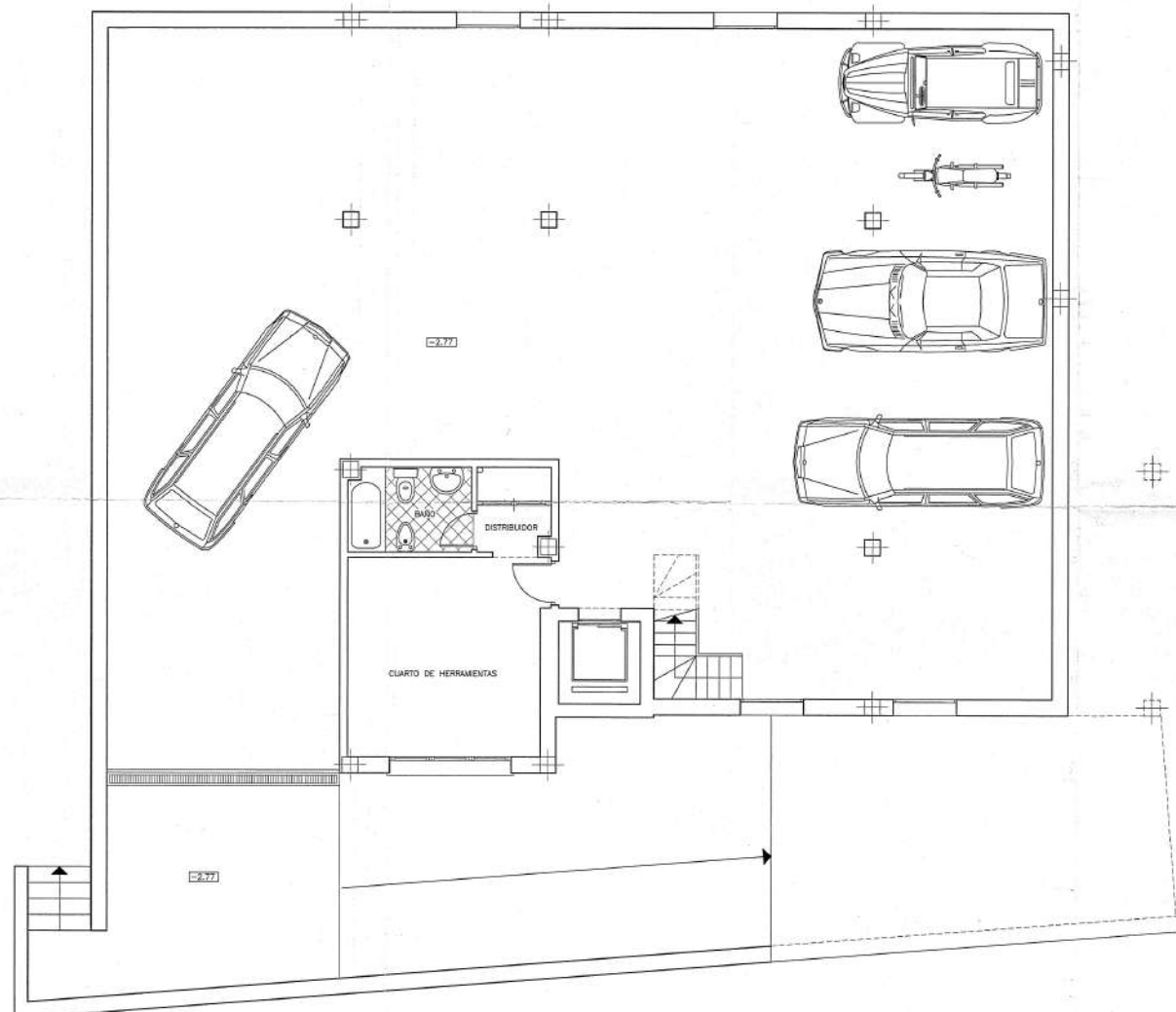
PLANTA SOTANO.-
