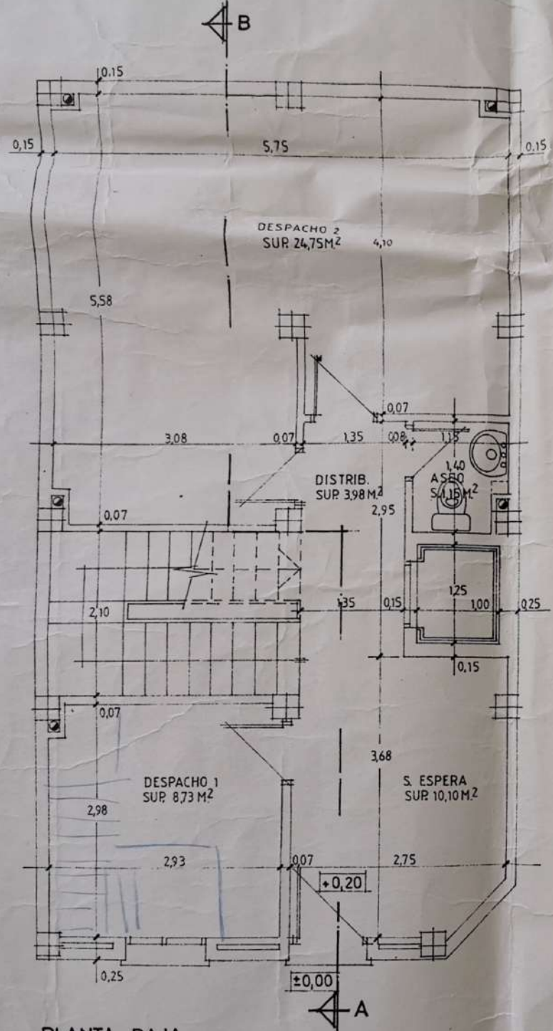
PLANTA BAJA
