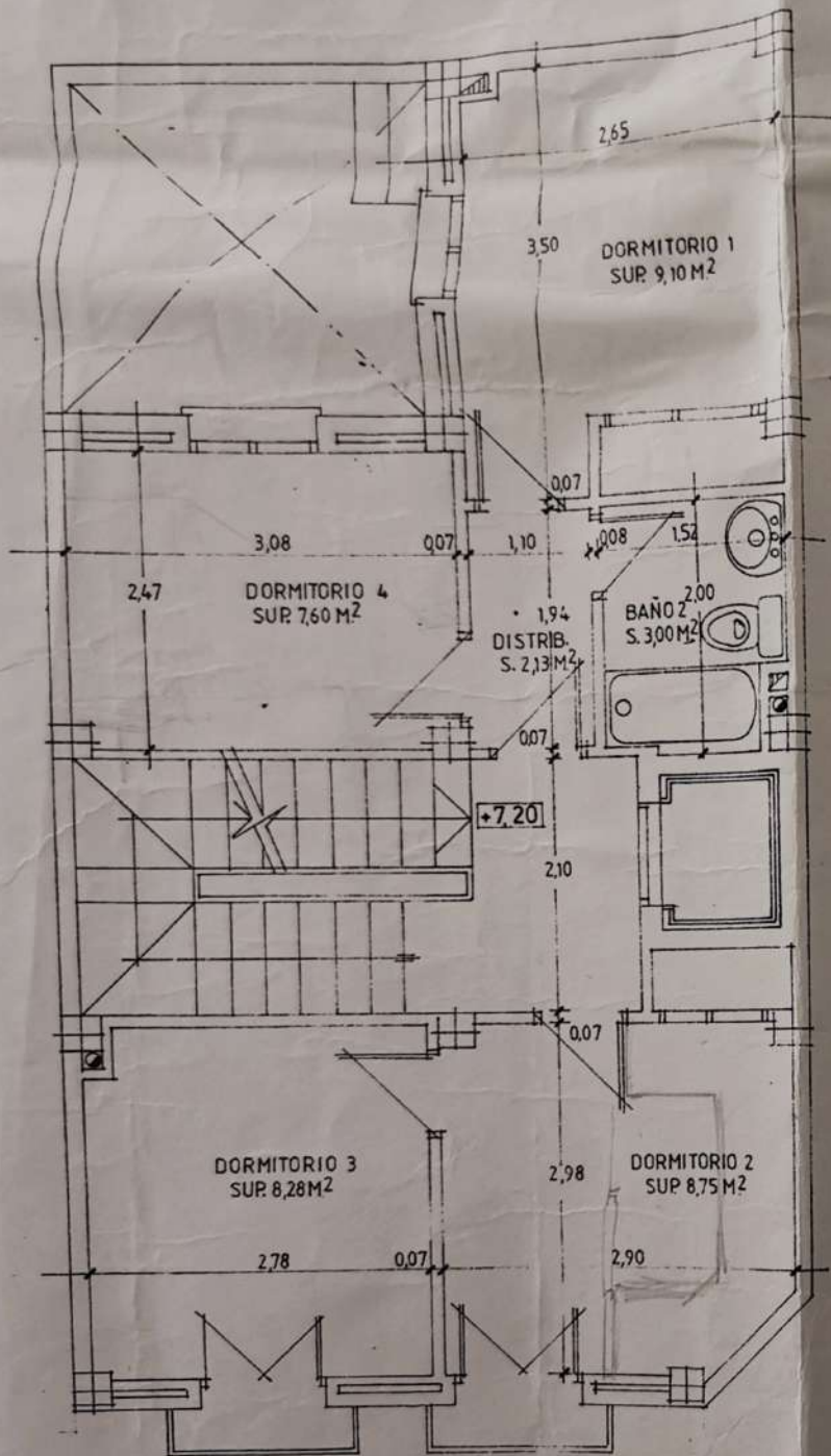
PLANTA SEGUNDA
