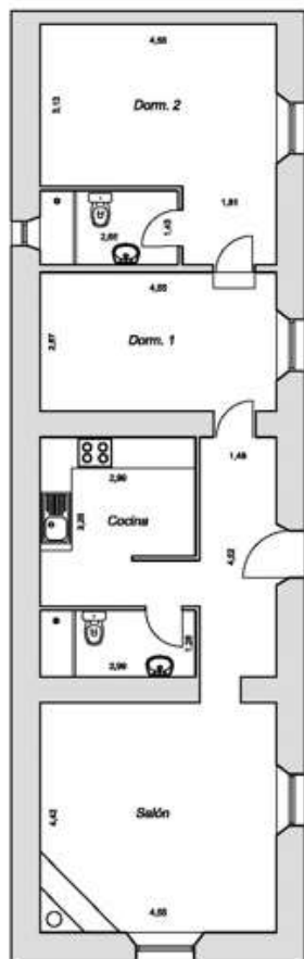
Planta Baja
