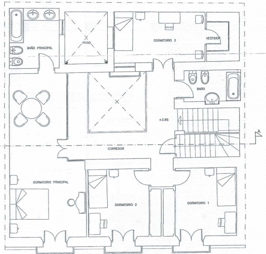
PLANTA PRIMERA
