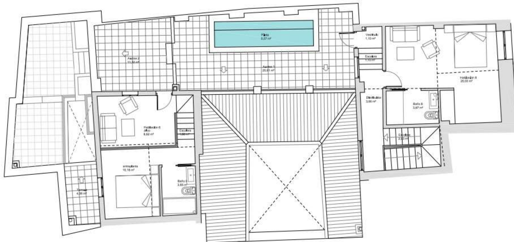
PLANTA SEGUNDA
