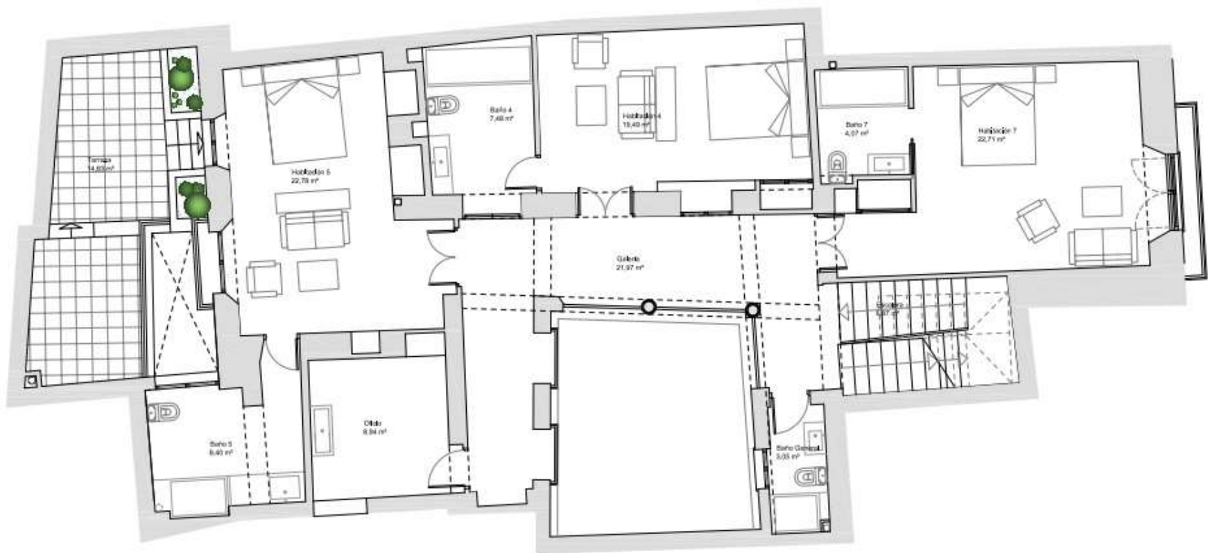
PLANTA PRIMERA
