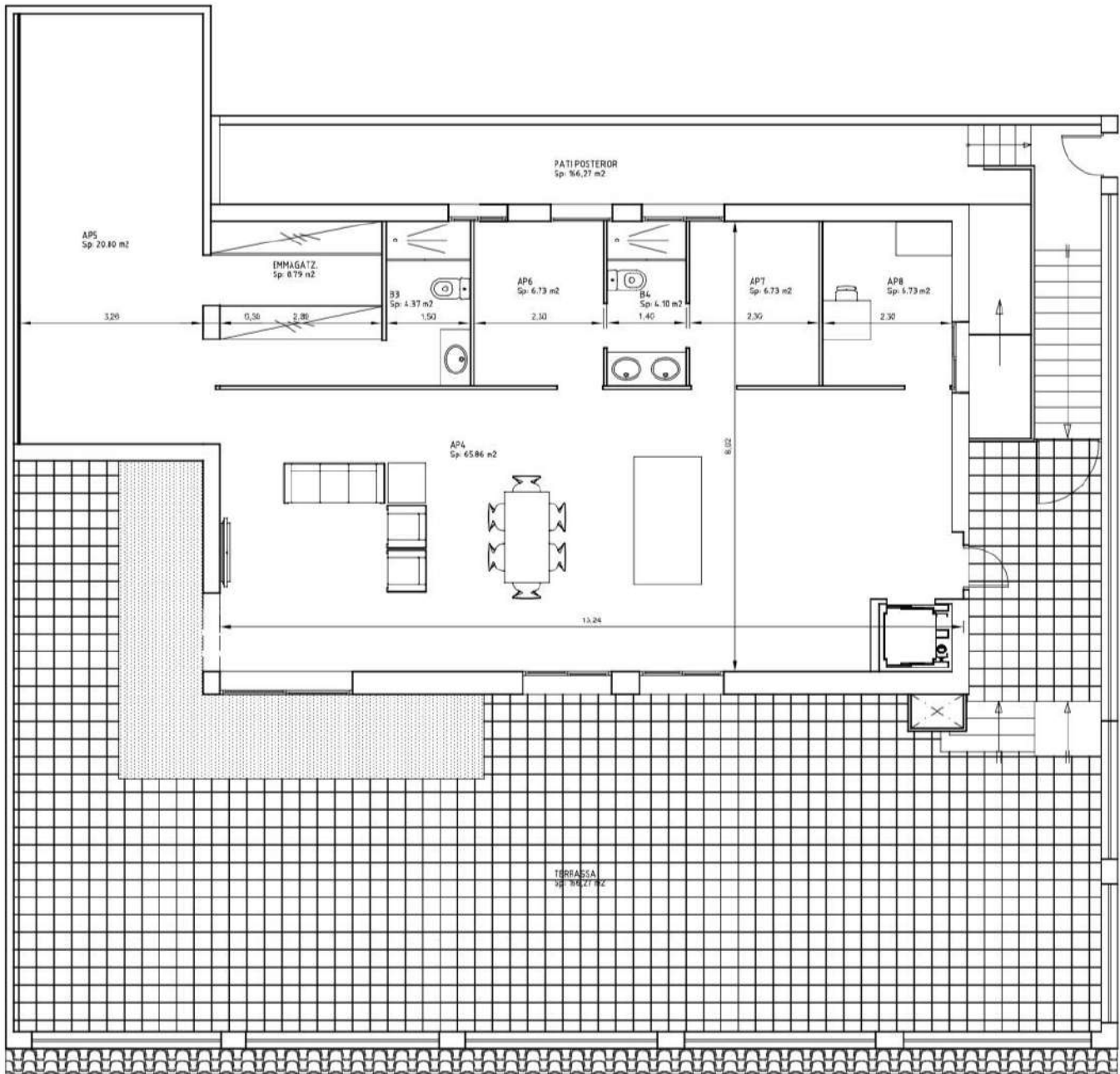
PLANTA PRIMERA PROJECTADA Esc. 1:100 Sup. Construida 147,90 m 2 .
