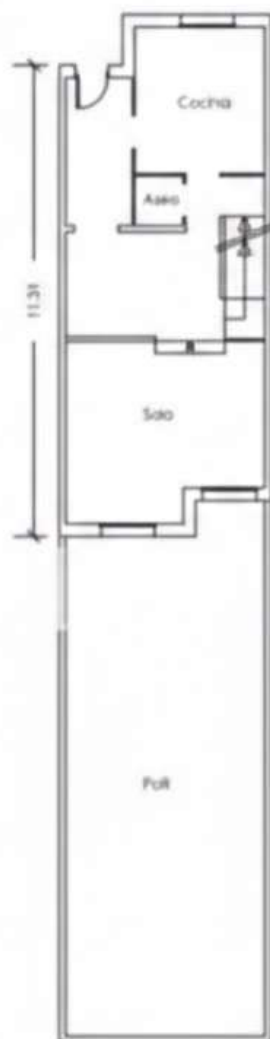
PLANTA BAJA
