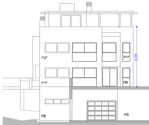
CASA UNO. ALZADO NORTE 1:100
