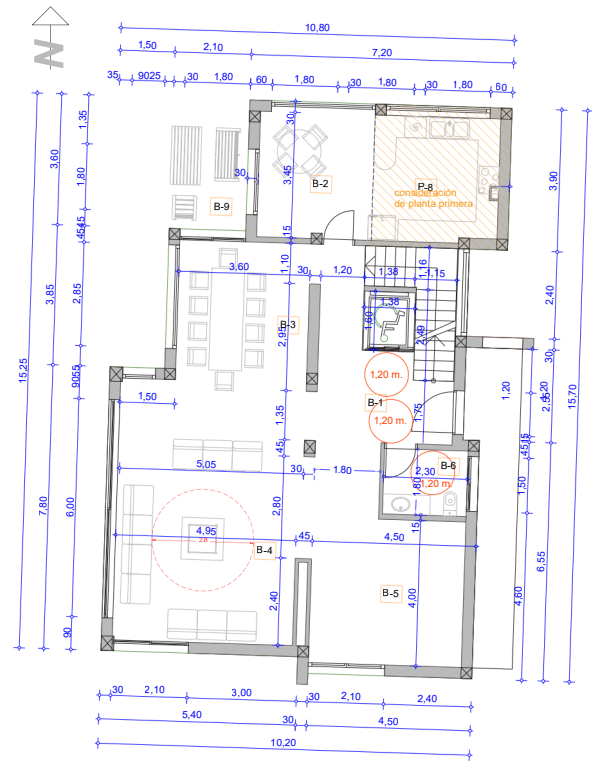
CASA UNO. PLANTA BAJA 1:100
