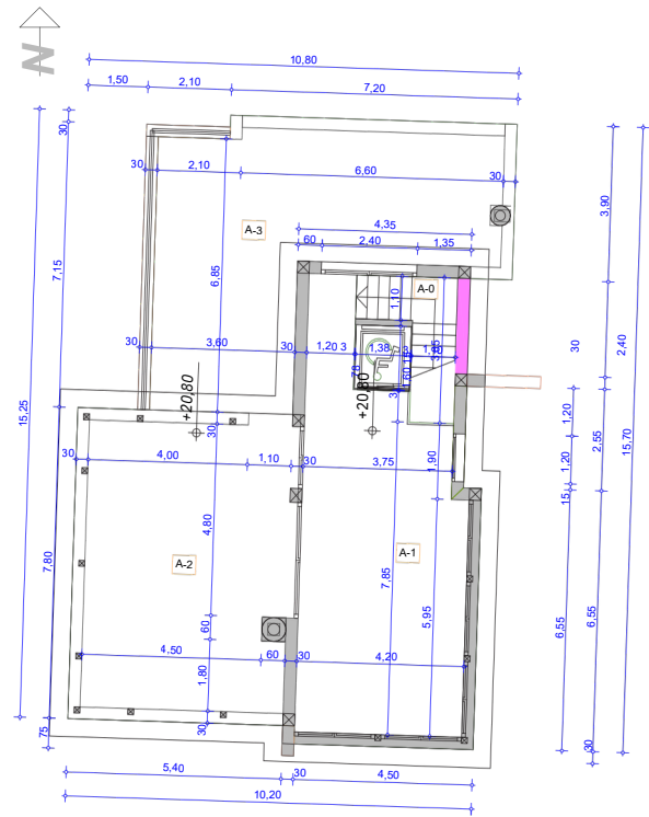
CASA UNO. PLANTA SEGUNDA 1:100
