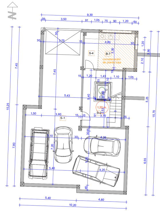
CASA UNO. PLANTA SOTANO 1:100
