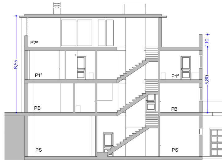
CASA UNO. SECCION LONGITUDINAL 1:100
