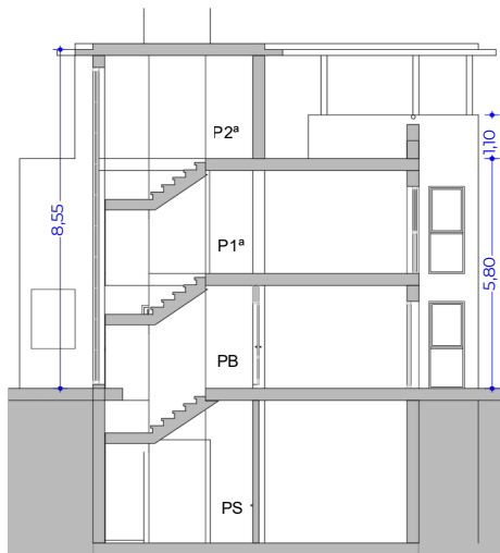
CASA UNO. SECCION TRANSVERSAL 1:100
