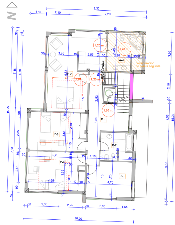
CASA UNO. PLANTA PRIMERA 1:100
