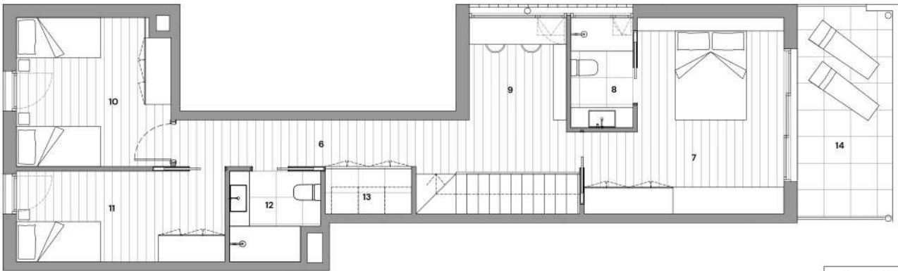
PLANTA PRIMERA (DÚPLEX 1)
