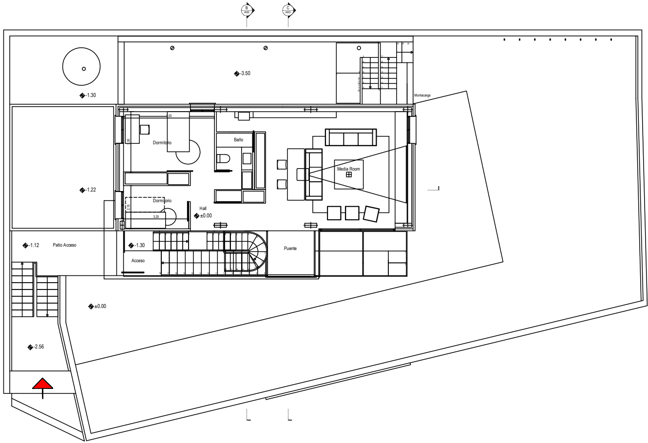
Planta 00
