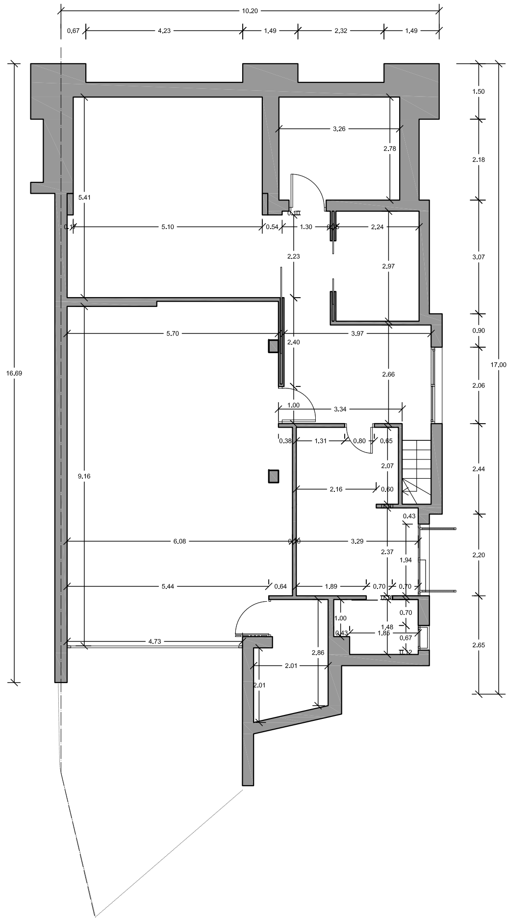
PLANTA SOTERRANI COTES
