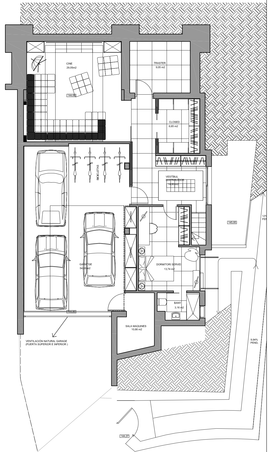
PLANTA SOTERRANI MOBILIARI
