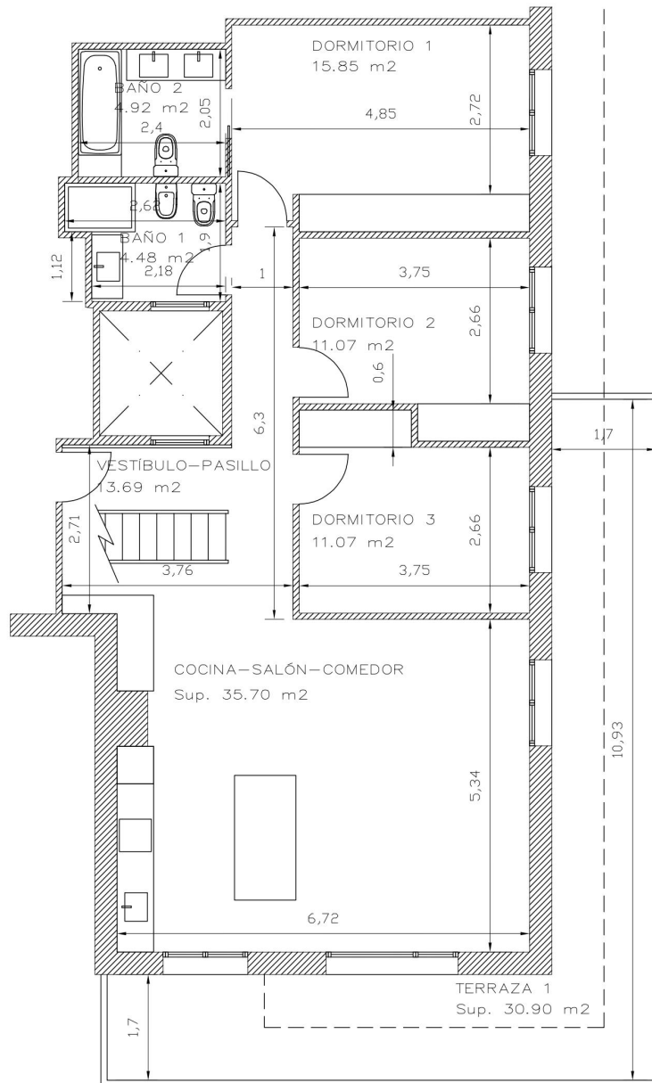
PLANTA 12 VIVIENDA
