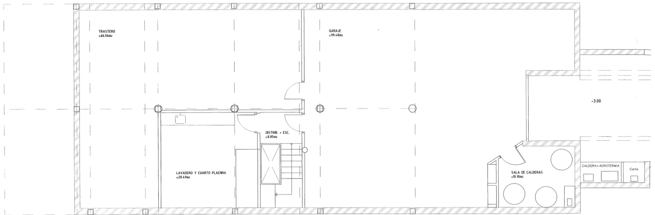
PLANTA SÓTANO
