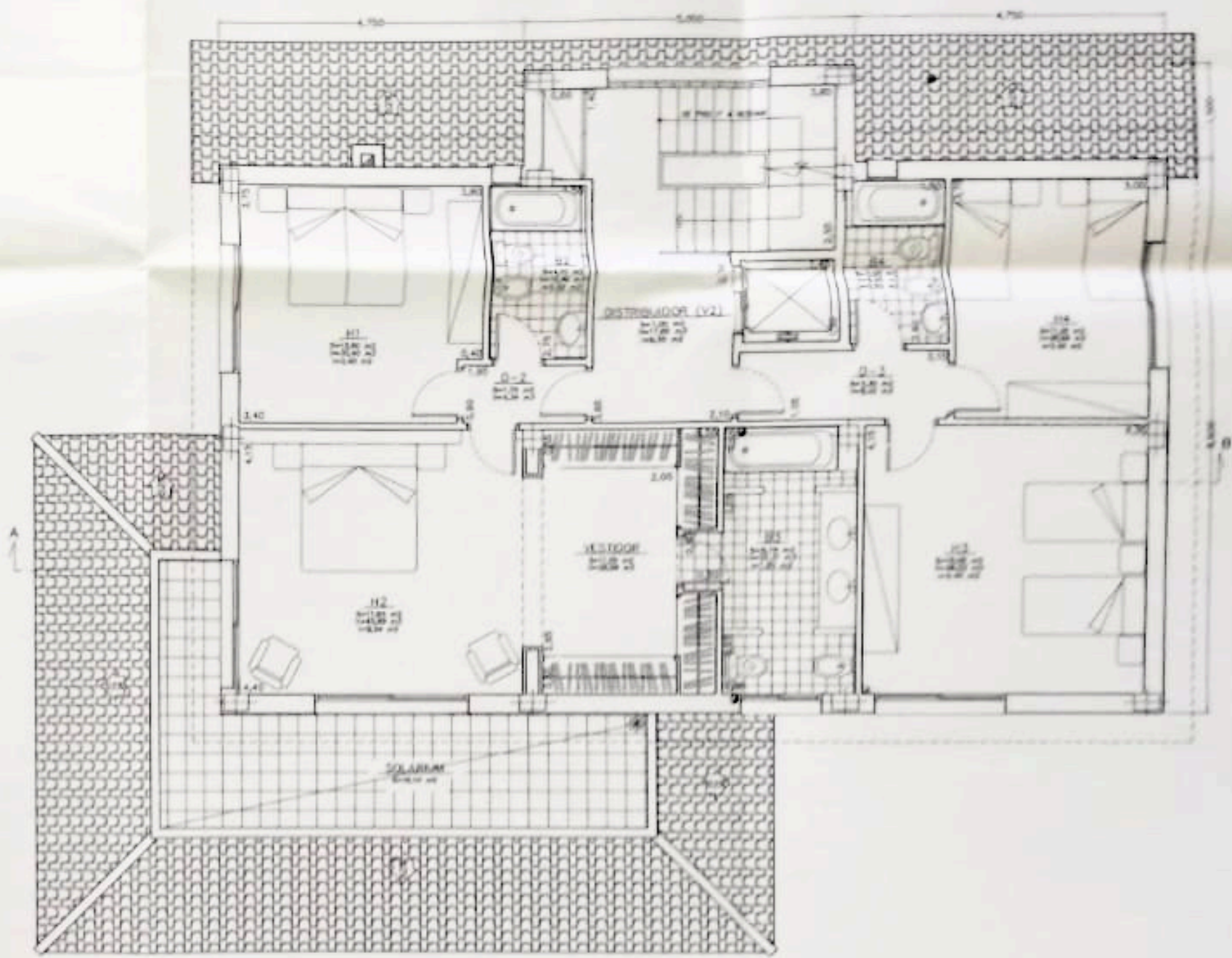
PLANTA PISO SUP. COTA. VIVIENDA: 132,85 m 2
