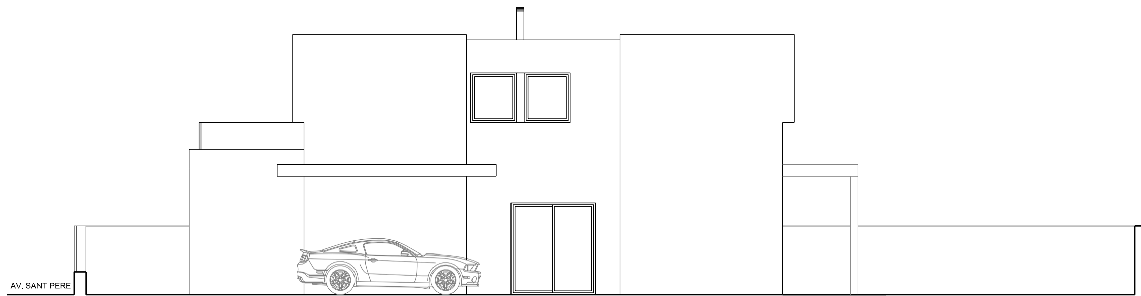
FAÇANA LATERAL 2
