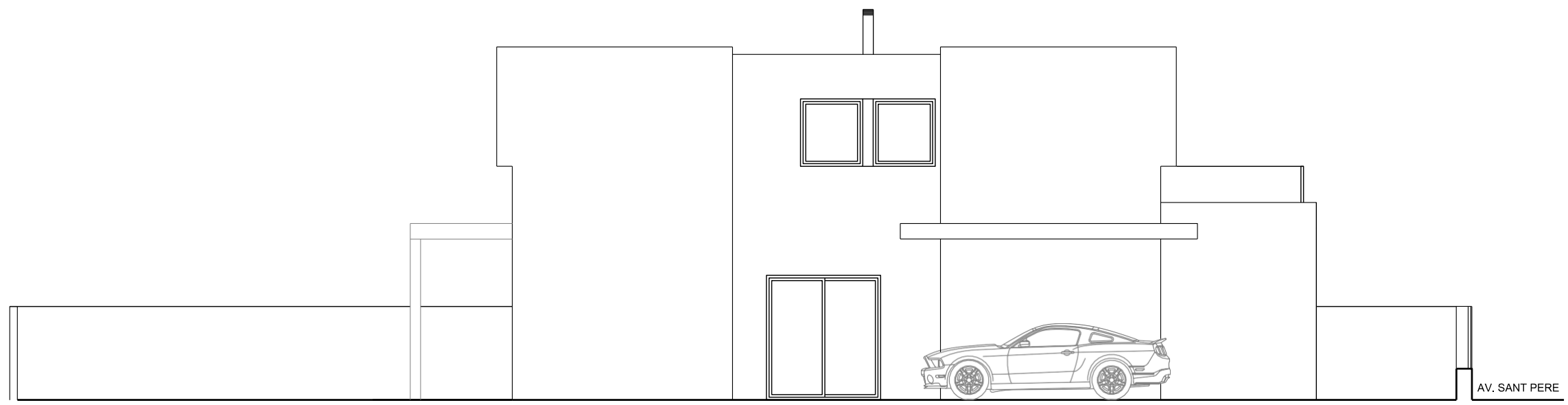
FAÇANA LATERAL 1
