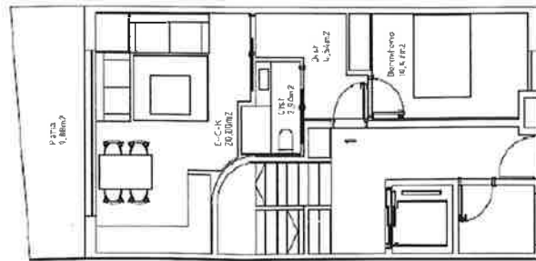
PLANTA BAJA ESPACIOS COMUNES VIVIENDA 1
