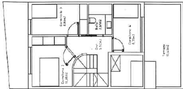
PLANTA ATICO ESPACIOS COMUNES VIVIENDA 4
