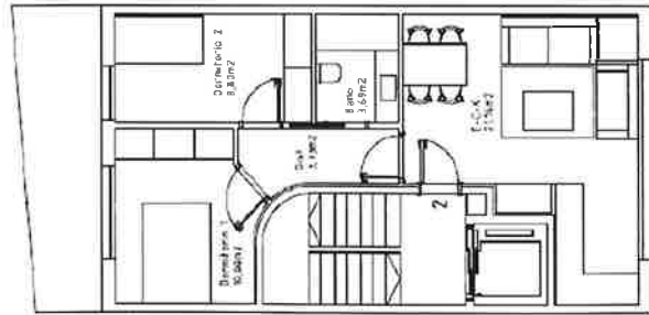
PLANTA PRIMERA ESPACIOS COMUNES VIVIENDA 2
