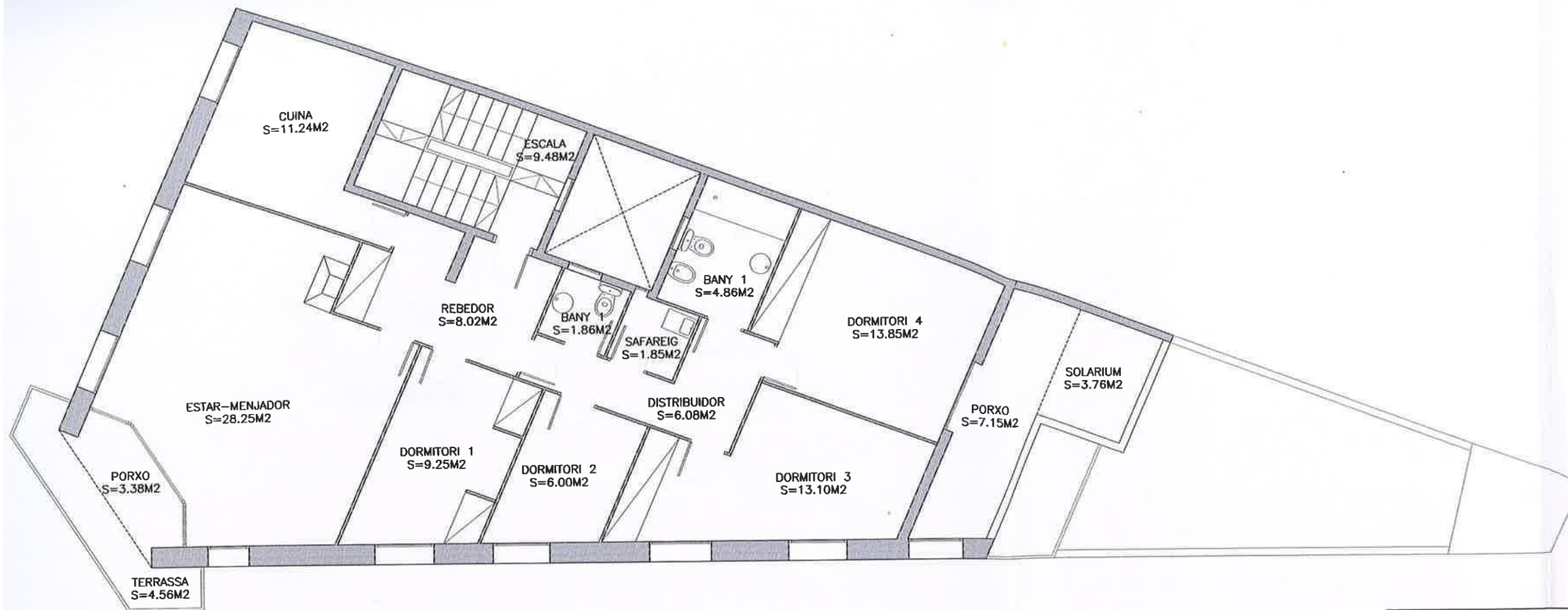
PLANTA TERCERA E:1/100
