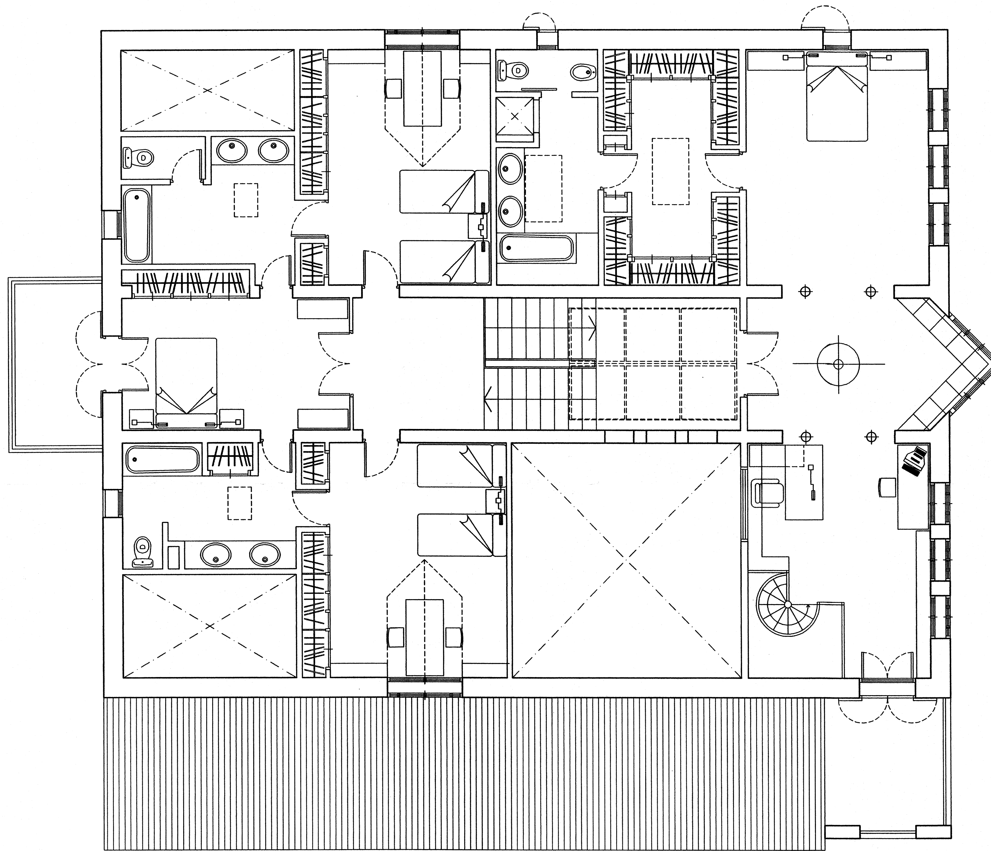
PLANTA PRIMERA ESCALA 1:50
