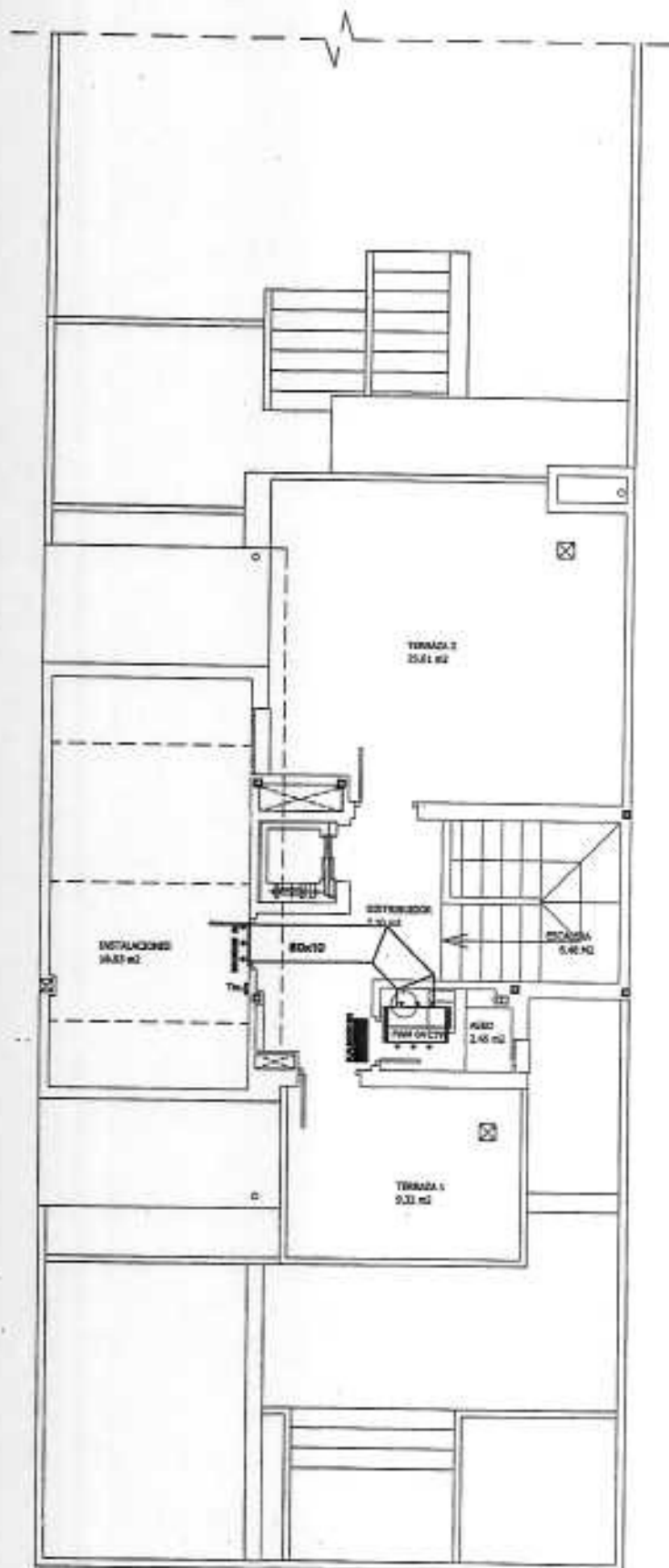
PLANTA ATICO
