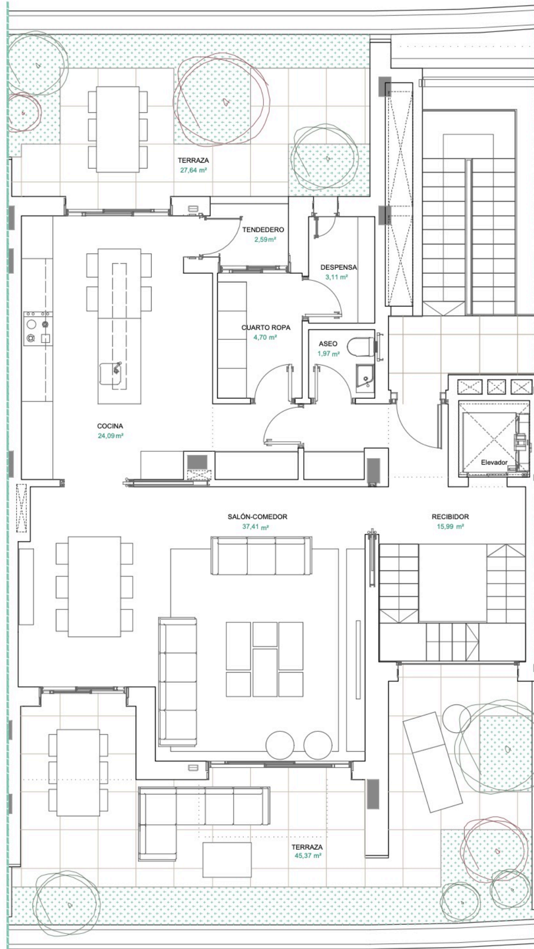
planta acceso vivienda con superficies útiles
