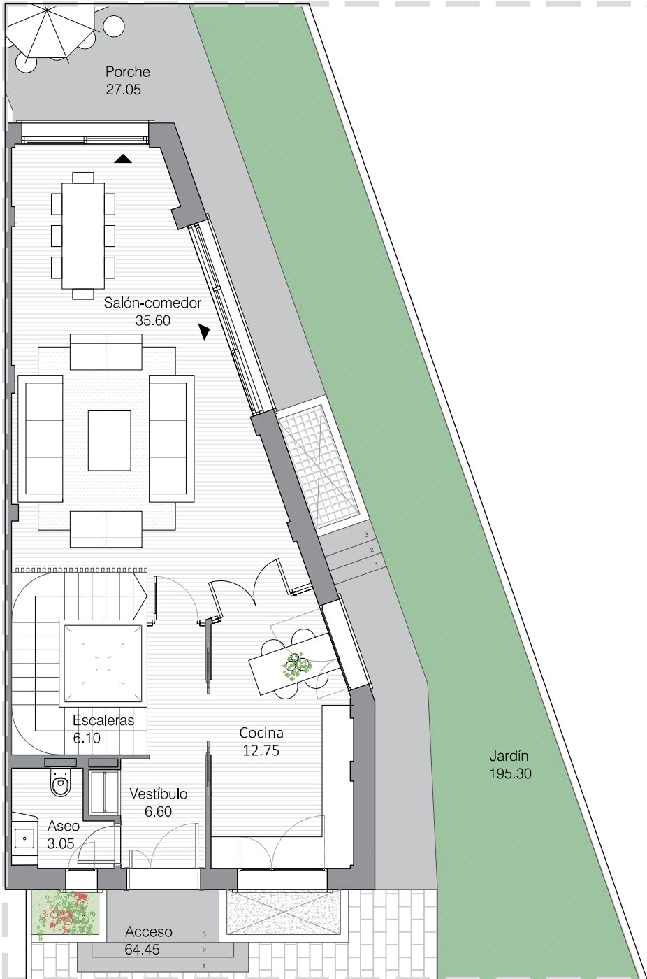
PLANTA BAJA
