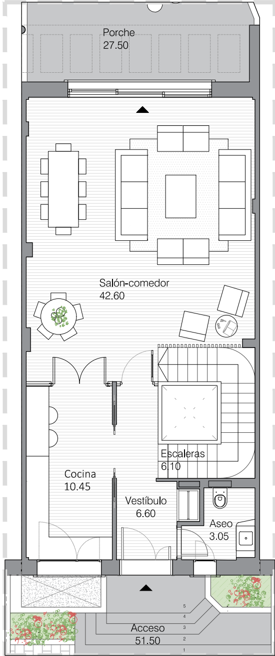
PLANTA BAJA
