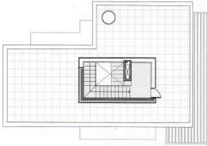
> PLANTA CASETÓN ACCESO_e: 1/150 proyecto licencia
