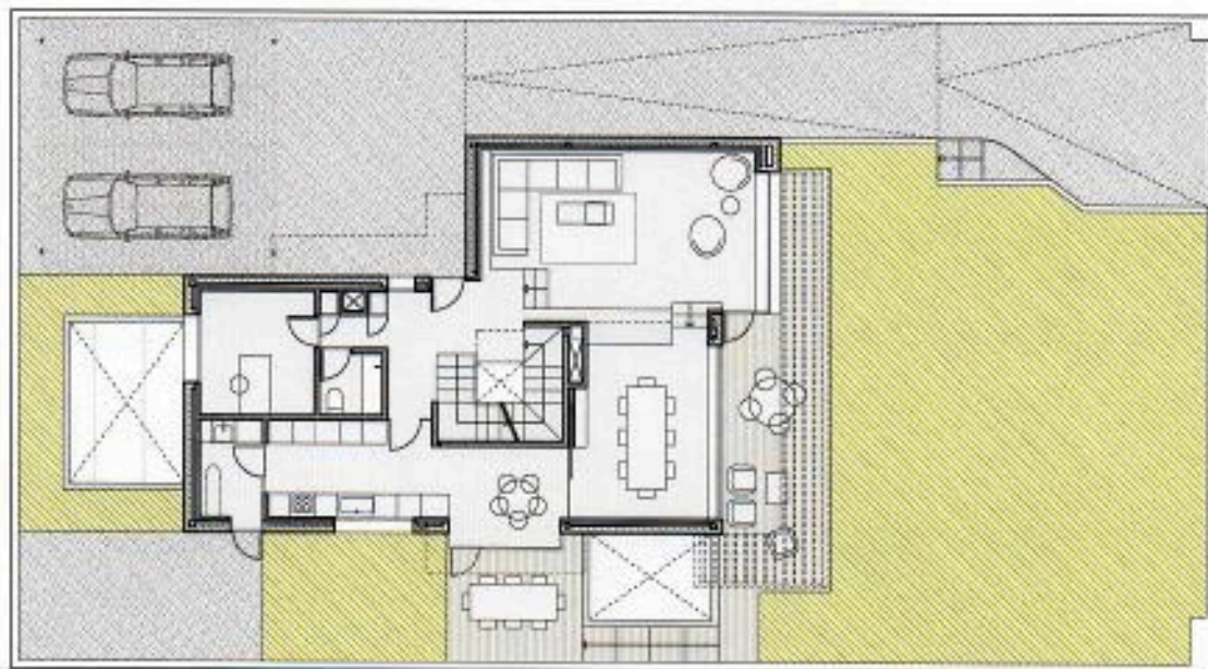
> PLANTA BAJA_e: 1/200 proyecto licencia
